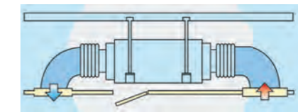
Забор воздуха с задней стороны блока
