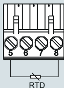
Двухпроводная система 1)
