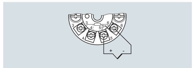
Термопары
