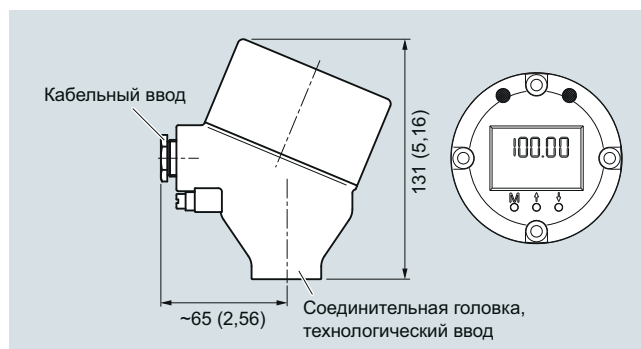
Соединительная головка с дисплеем 4—20 мА, алюминий, тип AN0, нержавеющая сталь, тип AV0, размеры в мм (дюймах)
