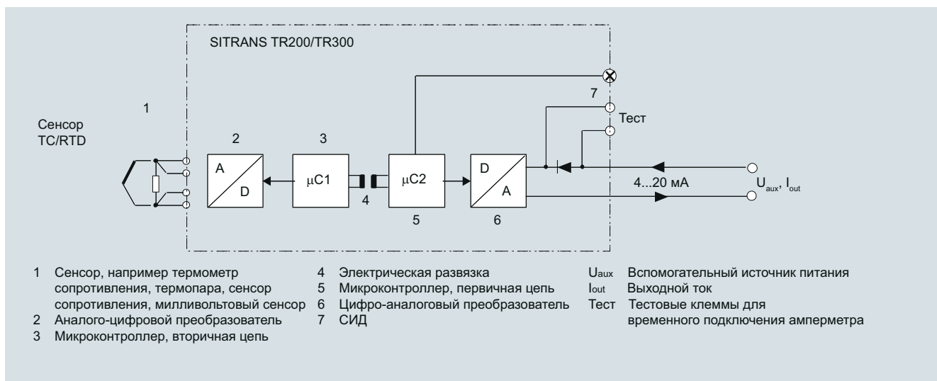
SITRANS TR300, функциональная схема
