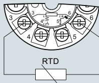
Двухпроводная система 1)
