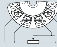
Четырехпроводная система
