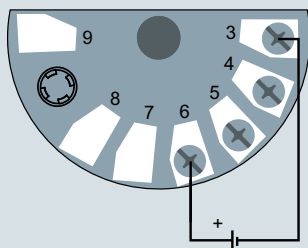
Вход напряжения (однополюсный или двухполюсный)
