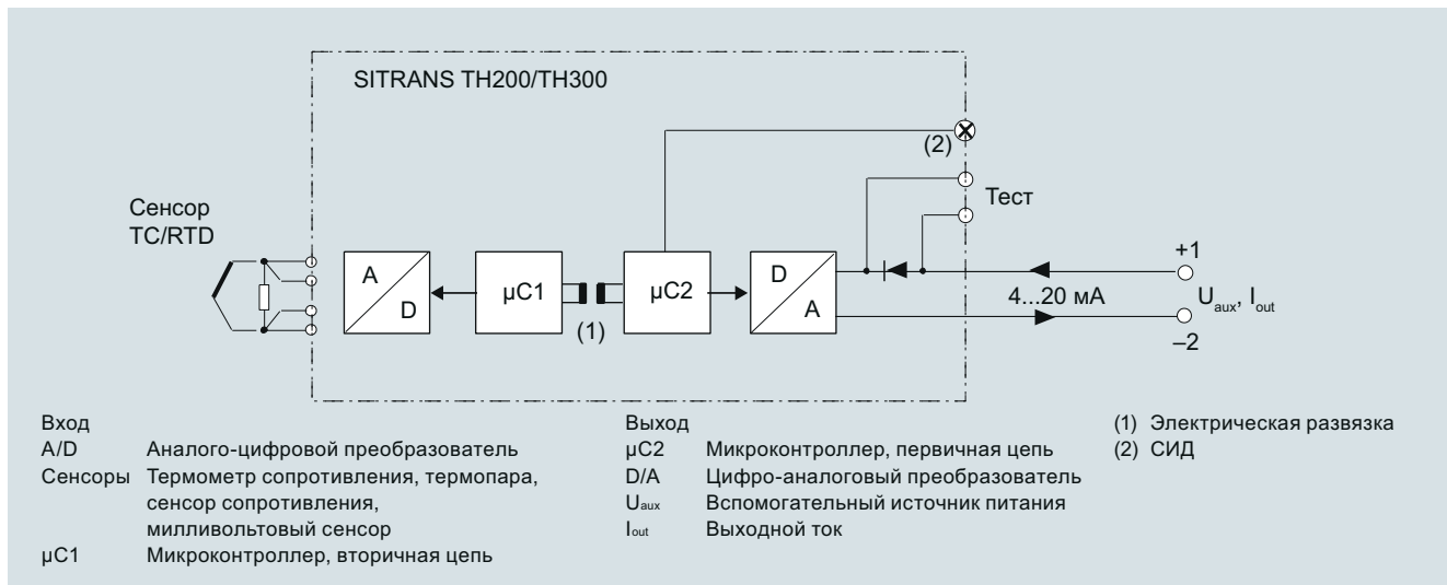
Функциональная схема SITRANS TH 300
