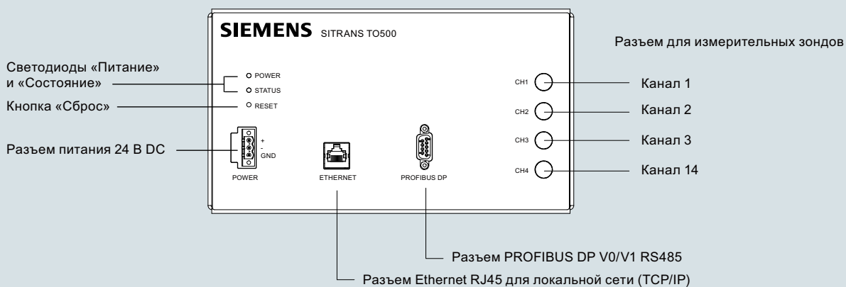
SITRANS TO500, назначение разъемов
