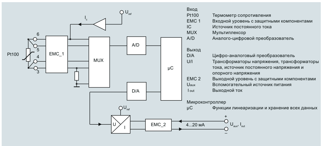
SITRANS TH100, функциональная схема
