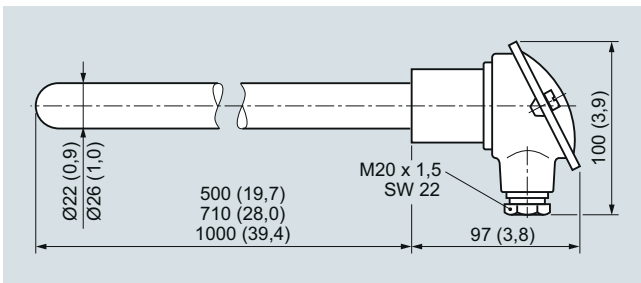
Прямая термопара, размеры в мм (дюймах)
