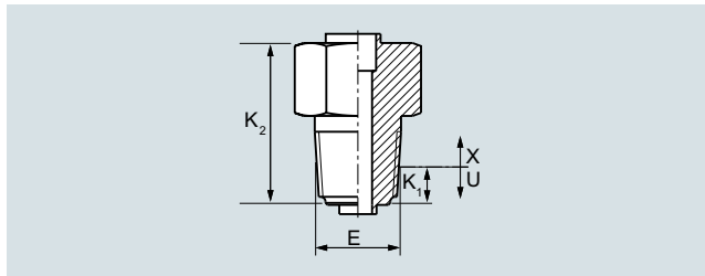
Резьба NPT
