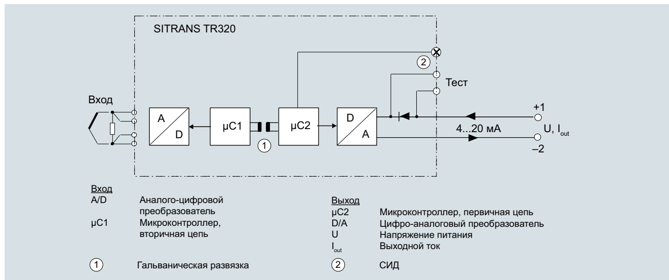
SITRANS TR320, функциональная блок-схема
