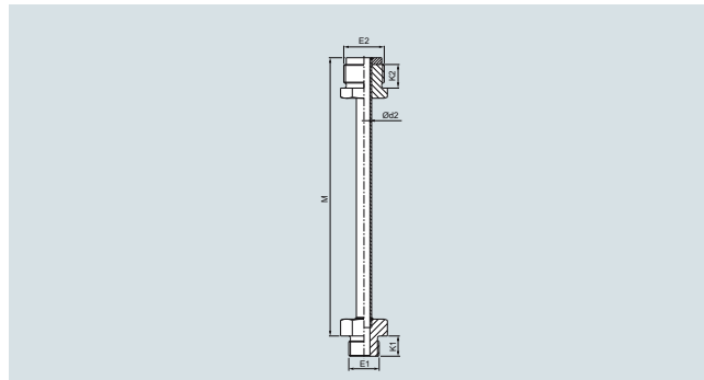
Удлинение (1, 2, 3), регулируемое, европейское, цилиндрическое, размеры в мм (дюймах)
