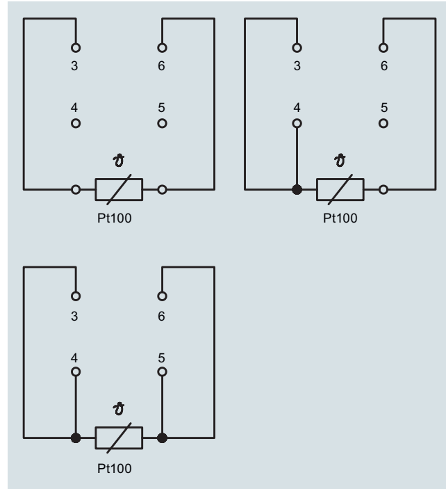
SITRANS TH100 Slim, назначение соединений сенсора
