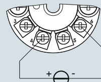
Один источник напряжения
