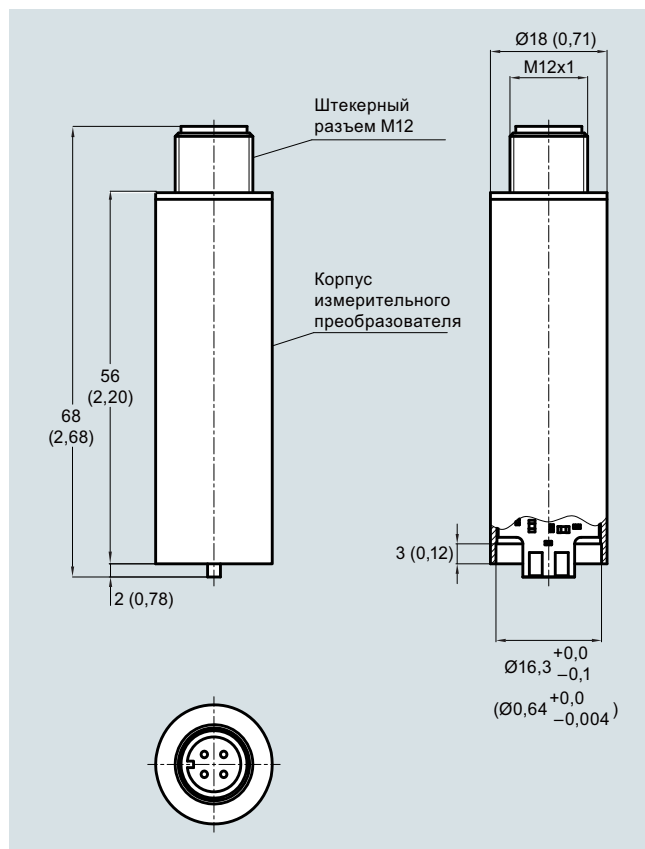
SITRANS TH100 Slim, размеры в мм (дюймах)
