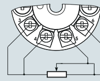
Четырехпроводная система
