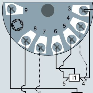
Вход 1 и/или вход 2: 3- или 4-проводной потенциометр
