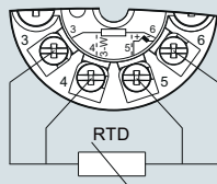
Четырехпроводная система
