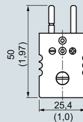
Разъем термопары, IP20, размеры в мм (дюймах)
