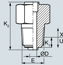
Коническое технологическое соединение, размеры в мм (дюймах)
