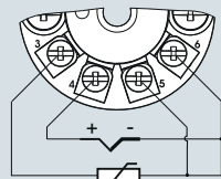
Компенсация холодного спая с внешним Pt100 в трехпроводной системе
