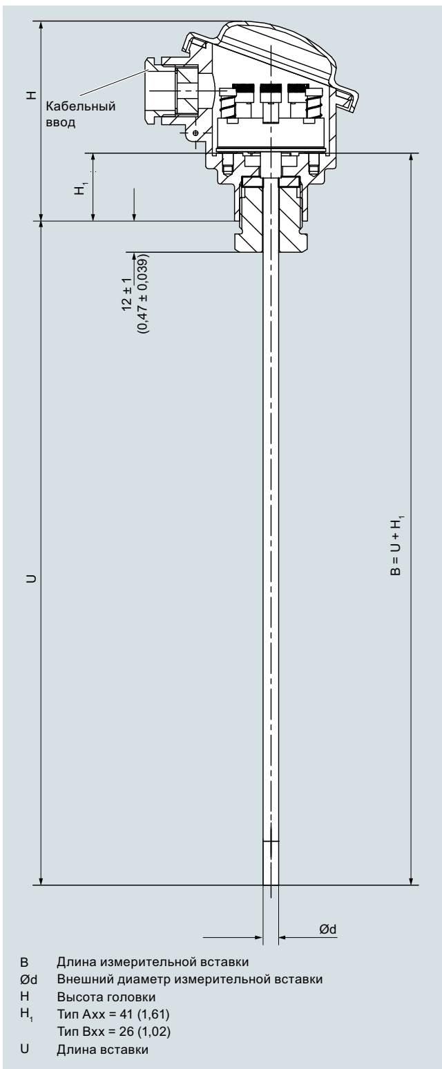
SITRANS TS500, опция G50 с уплотнением, ввод соединительной головки M24x1,5, размеры в мм (дюймах)
