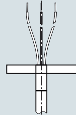
Проводные выводы, IP00, размеры в мм (дюймах)
