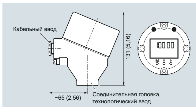
Соединительная головка с дисплеем 4—20 мА, алюминий, тип AH0, нержавеющая сталь, тип AV0, размеры в мм (дюймах)
