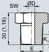
Припаяваемый штуцер, NPT (A22), размеры в мм (дюймах)
