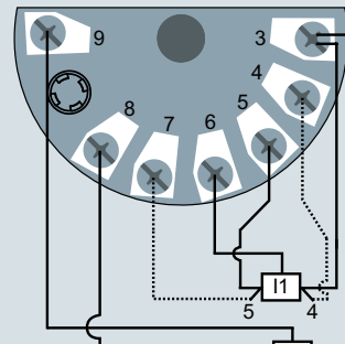
Вход 1: 5-проводной потенциометр Вход 2: 3-проводной потенциометр
