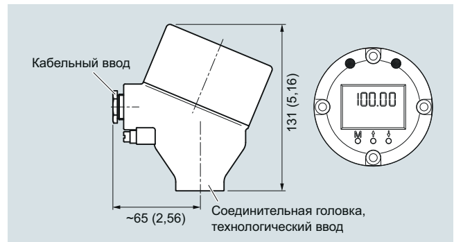
Соединительная головка с дисплеем 4—20 мА, алюминий, тип AH0, нержавеющая сталь, тип AV0, размеры в мм (дюймах)
