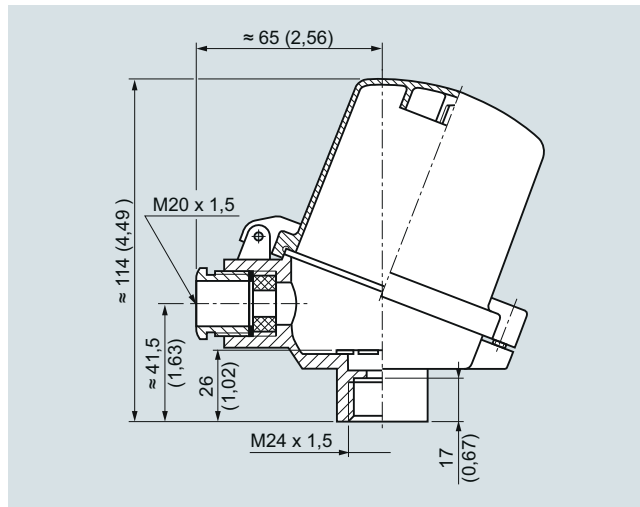
Соединительная головка, тип В, степень защиты IP65, из алюминия, с высокой откидной крышкой, размеры в мм (дюймах)
