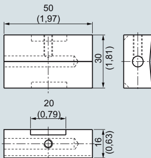
Элемент для соединения с поверхностью (A50), размеры в мм (дюймах)
