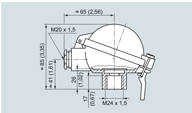
Соединительная головка, тип В, степень защиты IP65, из алюминия, со стандартной откидной крышкой, размеры в мм (дюймах)
