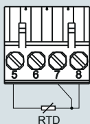
Трехпроводная система
