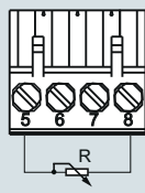
Двухпроводная система 1)
