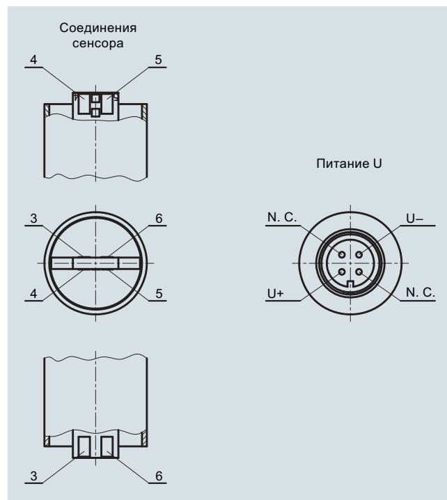
SITRANS TH100 Slim, соединение вспомогательного питания и сенсора
