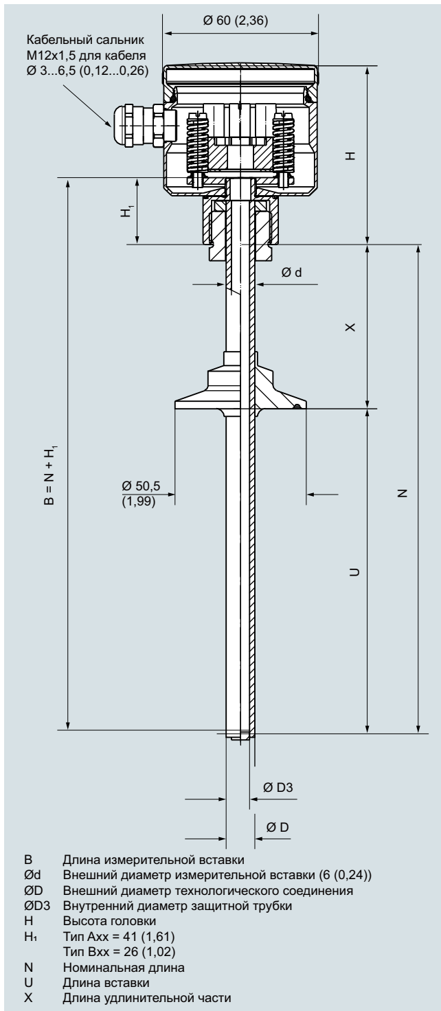
SITRANS TS300, модульная конструкция, размеры в мм (дюймах)
