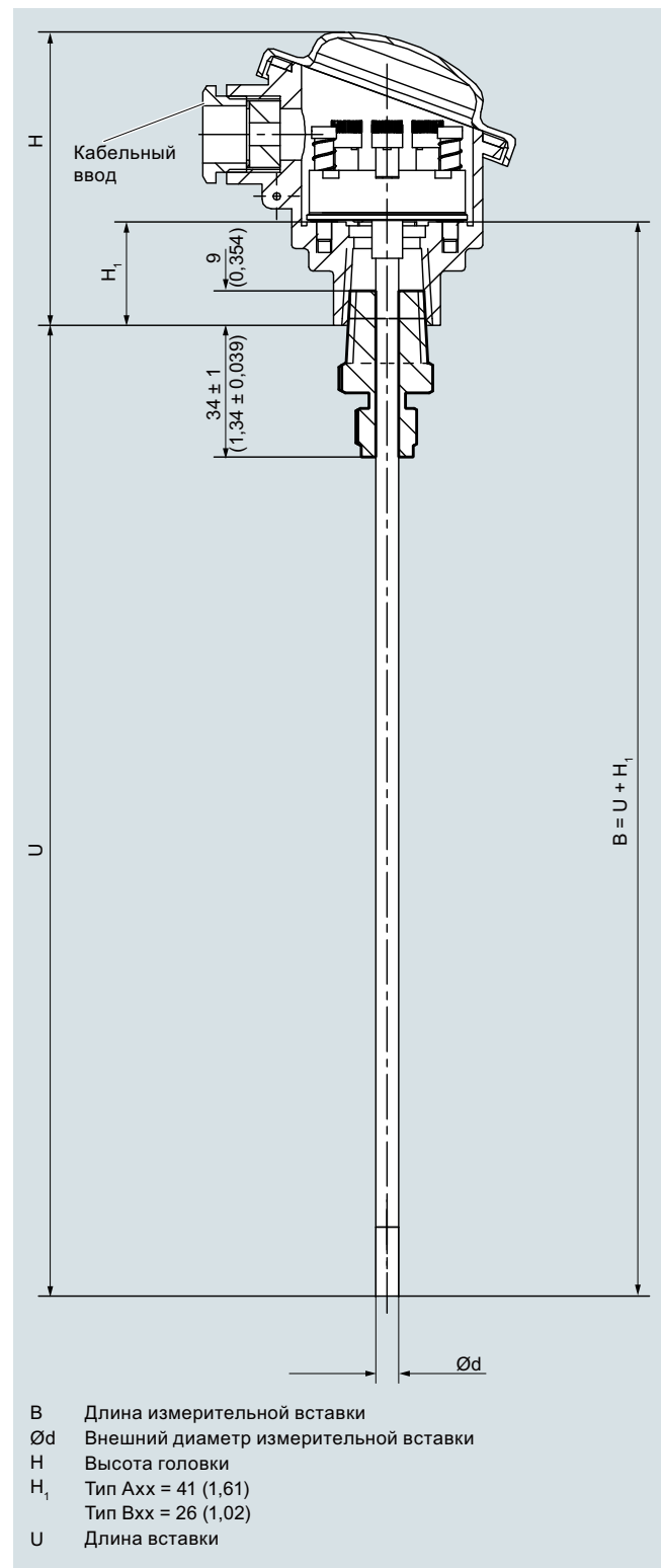
SITRANS TS500, опция G51 с уплотнением, ввод соединительной головки: ½" NPT, размеры в мм (дюймах)
