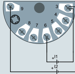
Вход 1 и/или вход 2: вход напряжения (однополюсный или двухполюсный)
