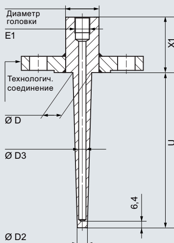
7MT43, фланцевое соединение, коническая
