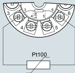
Двухпроводная система (настраиваемое линейное сопротивление)
