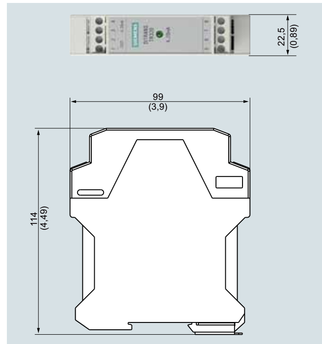
SITRANS TR320, размеры в мм (дюймах)
