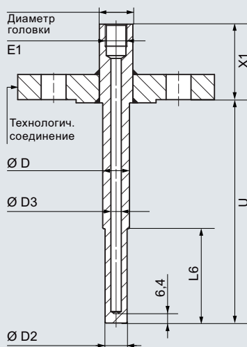
7MT43, фланцевое соединение, коническая
