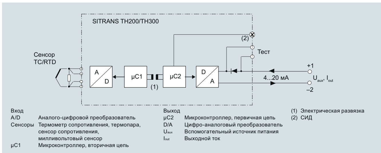
Функциональная схема SITRANS TH200
