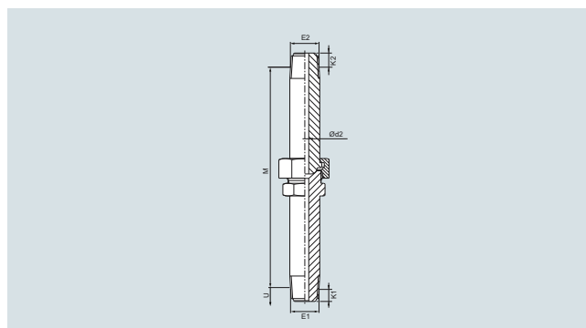
Удлинение NUN, регулируемое, коническое, европейское (5), американское (8), размеры в мм (дюймах)
