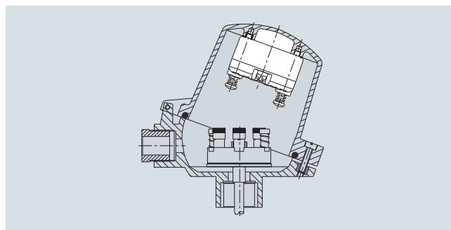
Установка с откидной крышкой
