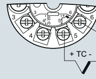
Компенсация холодного спая Внутренняя / фиксированное значение
