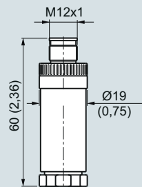
Штекерный разъем M12, IP54, размеры в мм (дюймах)
