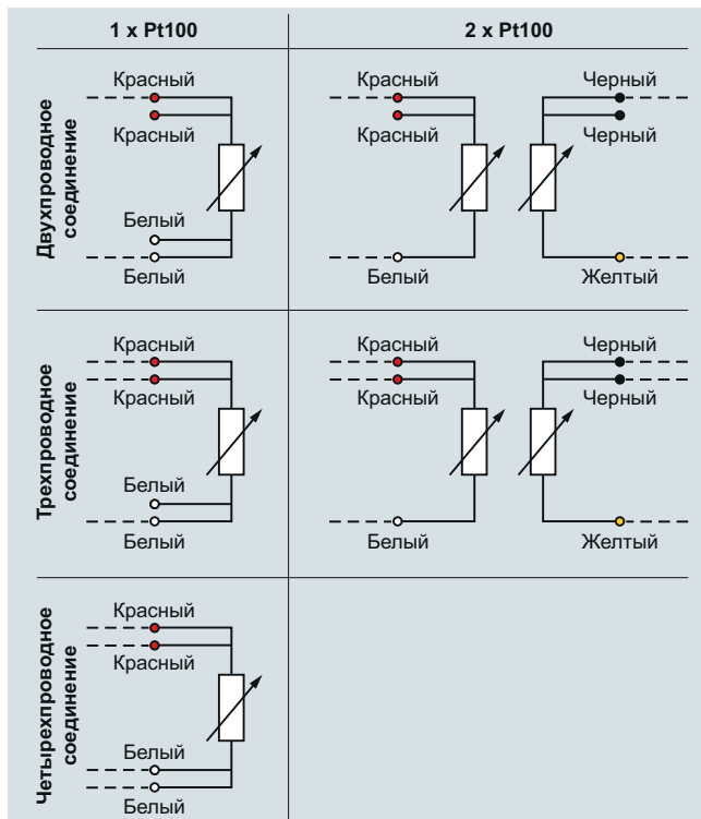
Схема от 1 × Pt100-2 Вт до 2 × Pt100-4 Вт
