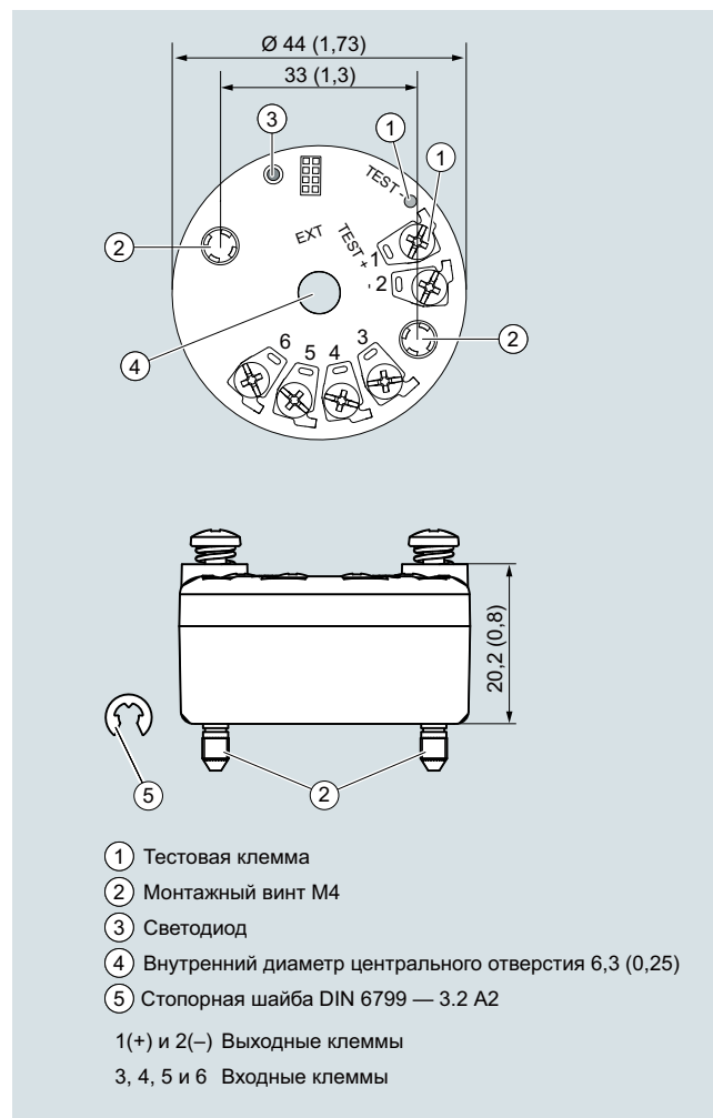
SITRANS TH320, размеры и назначение контактов, размеры в мм (дюймах)
