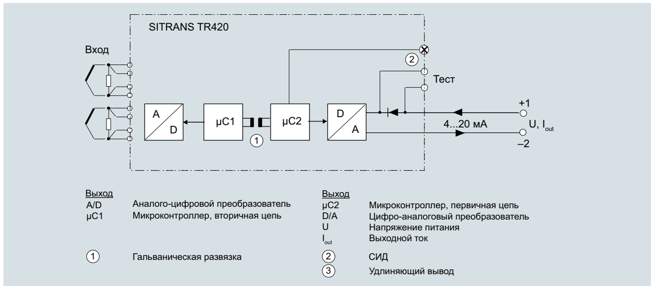
SITRANS TR420, функциональная блок-схема
