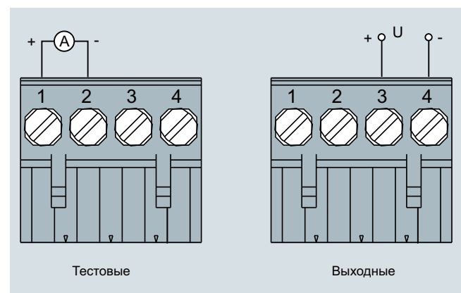
SITRANS TR420, назначение соединений выхода
