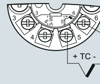
Компенсация холодного спая Внутренняя / фиксированное значение
