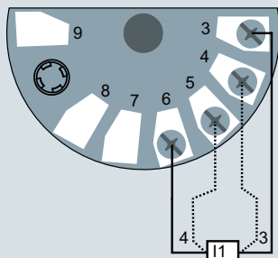
2-, 3- или 4-проводной RTD или линейное сопротивление
