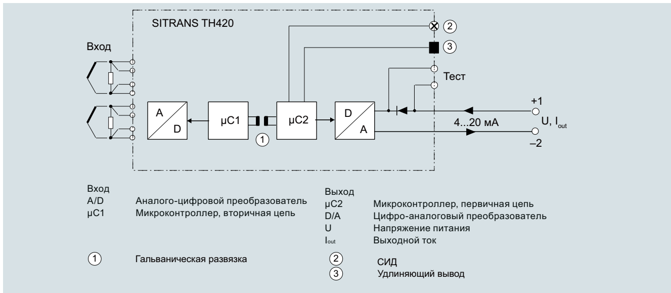
SITRANS TH420, функциональная блок-схема
