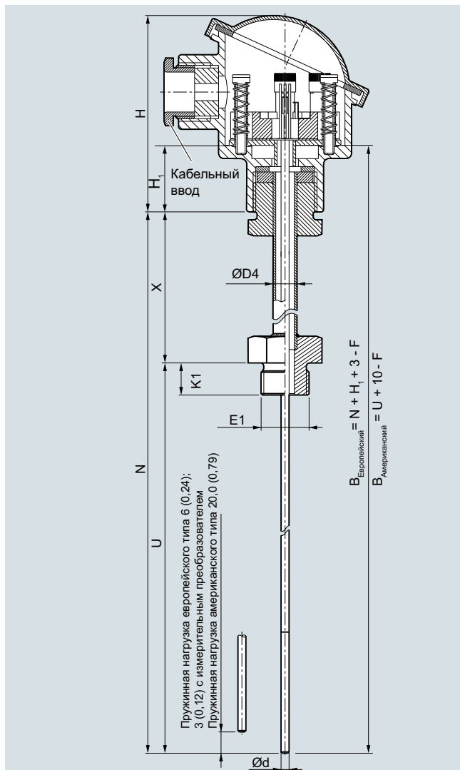
Удлинение (1, 2, 3), регулируемое, европейское, цилиндрическое, размеры в мм (дюймах)
