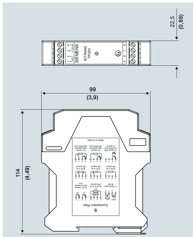
SITRANS TR300, размеры в мм (дюймах)
