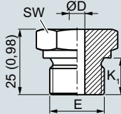
Припаяваемый штуцер, метрический (A20, A21, A23), размеры в мм (дюймах)
