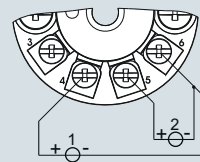
Измерение среднего значения, разности и резервирование с 2 источниками напряжения
