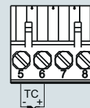
Компенсация холодного спая внутренняя / фиксированное значение
