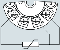
Трехпроводная система
