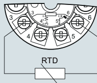
Двухпроводная система 1)
