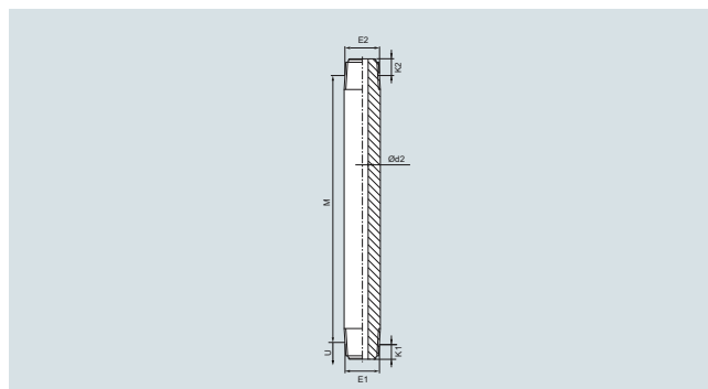
Удлинение, штуцер, нерегулируемое, коническое, европейское (4), американское (6), размеры в мм (дюймах)
