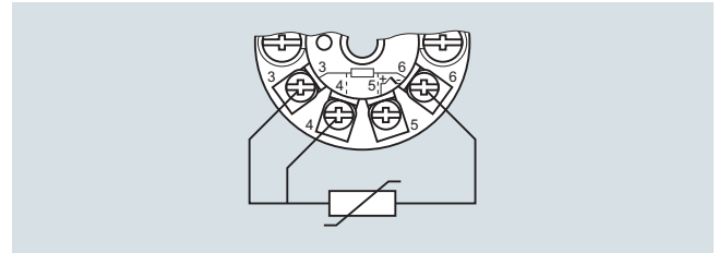
Термометр сопротивления
