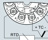
Компенсация холодного спая с внешним Pt100 в двухпроводной системе 1)
