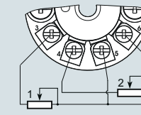
Формирование усредненного/дифференциального значения или резервирование и компенсация холодного спая с внутренним Pt100 в двухпроводной системе 1)
