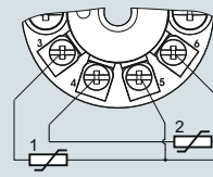
Формирование усредненного/дифференциального значения или резервирование, 1 сенсор в двухпроводной системе 1) , 1 сенсор в трехпроводной системе
