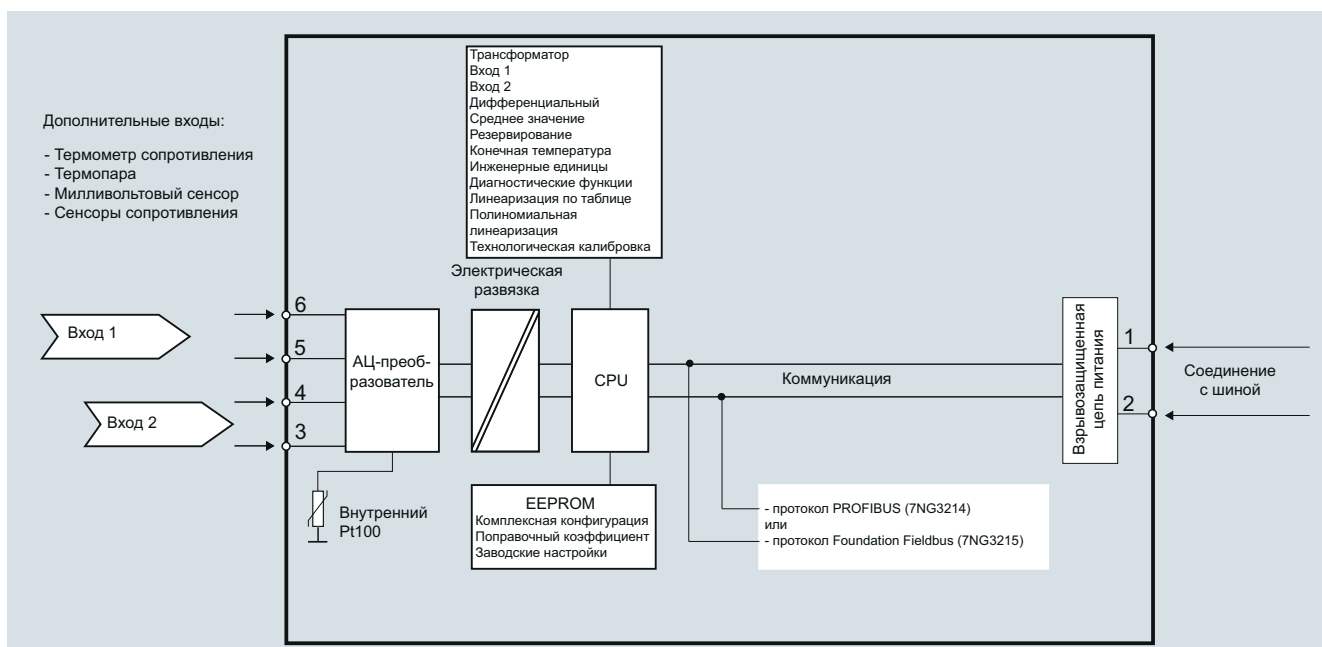
SITRANS TH400, функциональная схема
