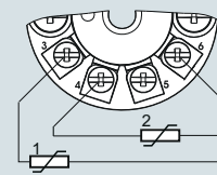
Формирование усредненного/дифференциального значения или резервирование 2 × двухпроводные системы 1)
