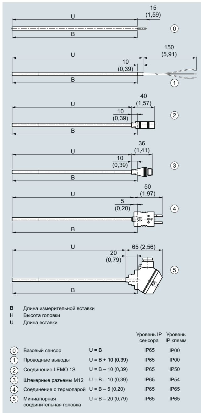
SITRANS TS100 с минеральной изоляцией (MIC) IP54 в месте соединения сенсора с кабелем, разъем — см. таблицу
