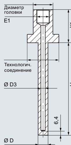
7MT52, тип со свободным соединением, суженная
