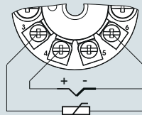
Компенсация холодного спая с внешним Pt100 в двухпроводной системе 1)
