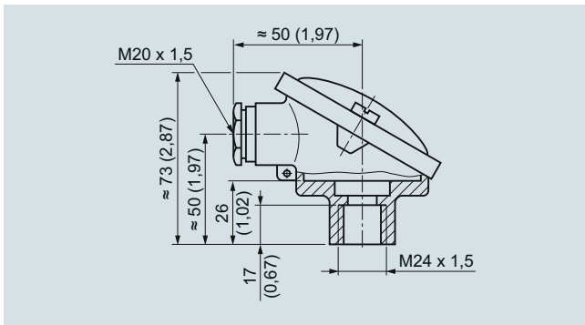
Соединительная головка, тип В, степень защиты IP54, из алюминия, с резьбовой крышкой, размеры в мм (дюймах)
