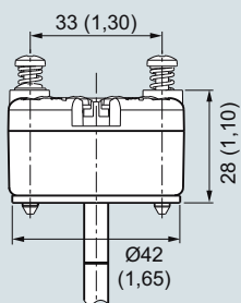
Европейский тип: с холодным концом, встроенный измерительный преобразователь, размеры в мм (дюймах)
