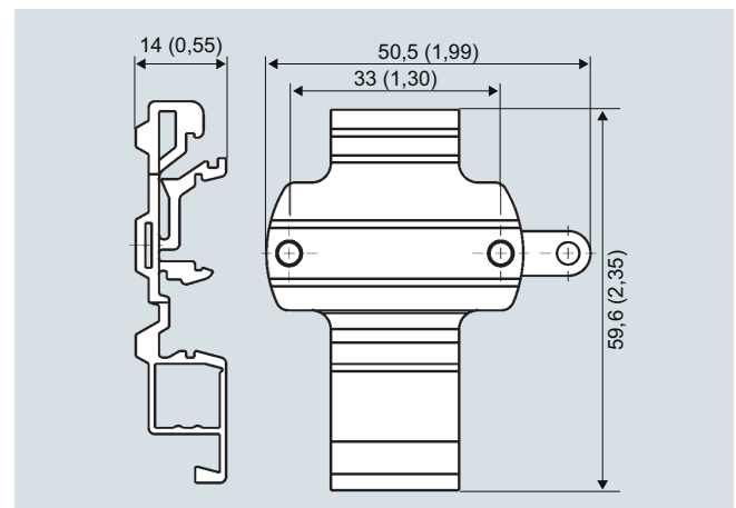
Переходник на DIN-рейку, размеры в мм (дюймах)
