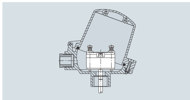
Установка с измерительной вставкой
