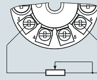
Двухпроводная система 1)
