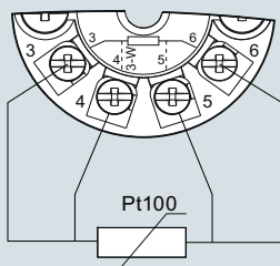
Четырехпроводная система
