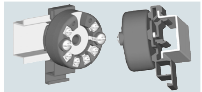
SITRANS TH100, монтаж измерительного преобразователя на DIN-рейку
