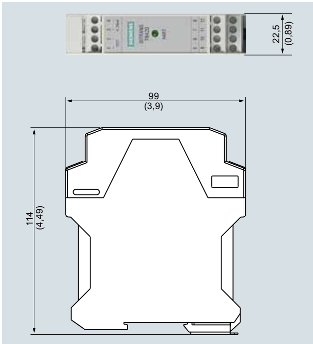
SITRANS TR420, размеры в мм (дюймах)
