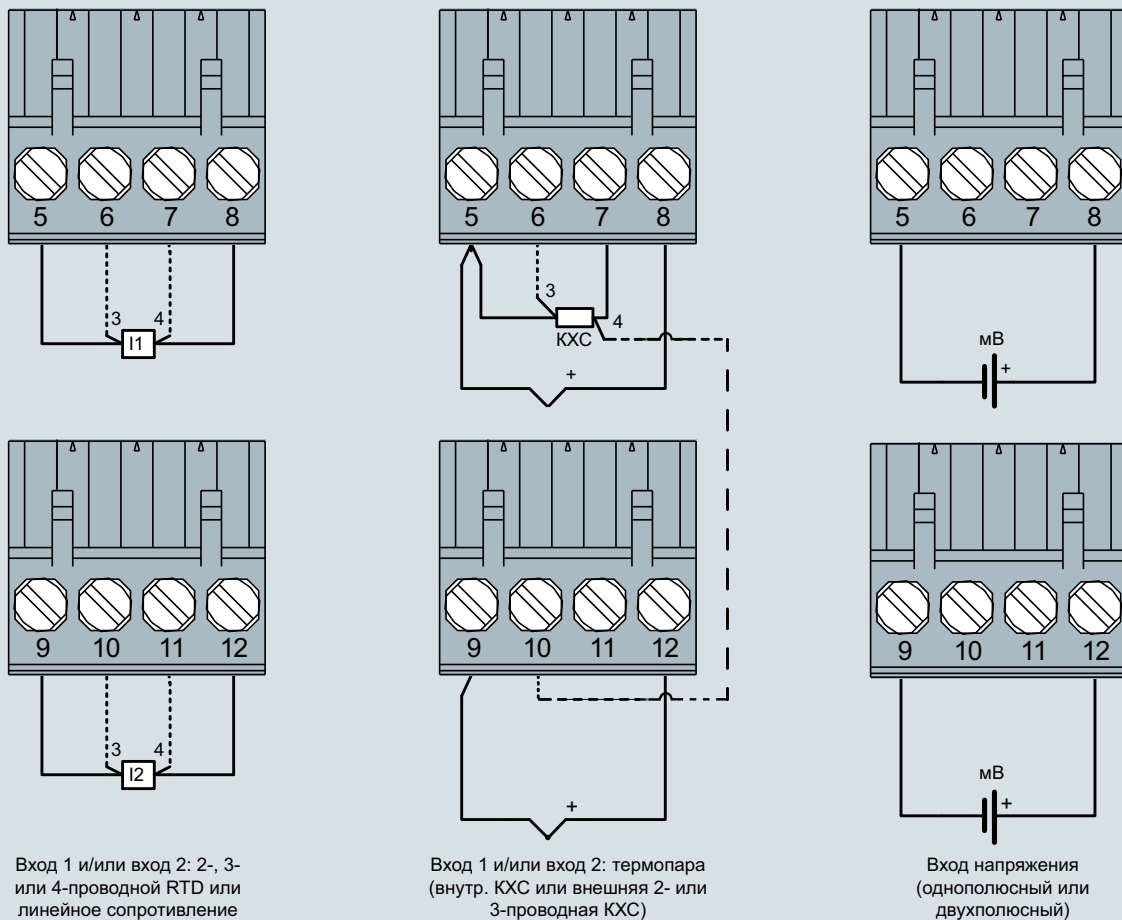
SITRANS TR420, назначение соединений входа
