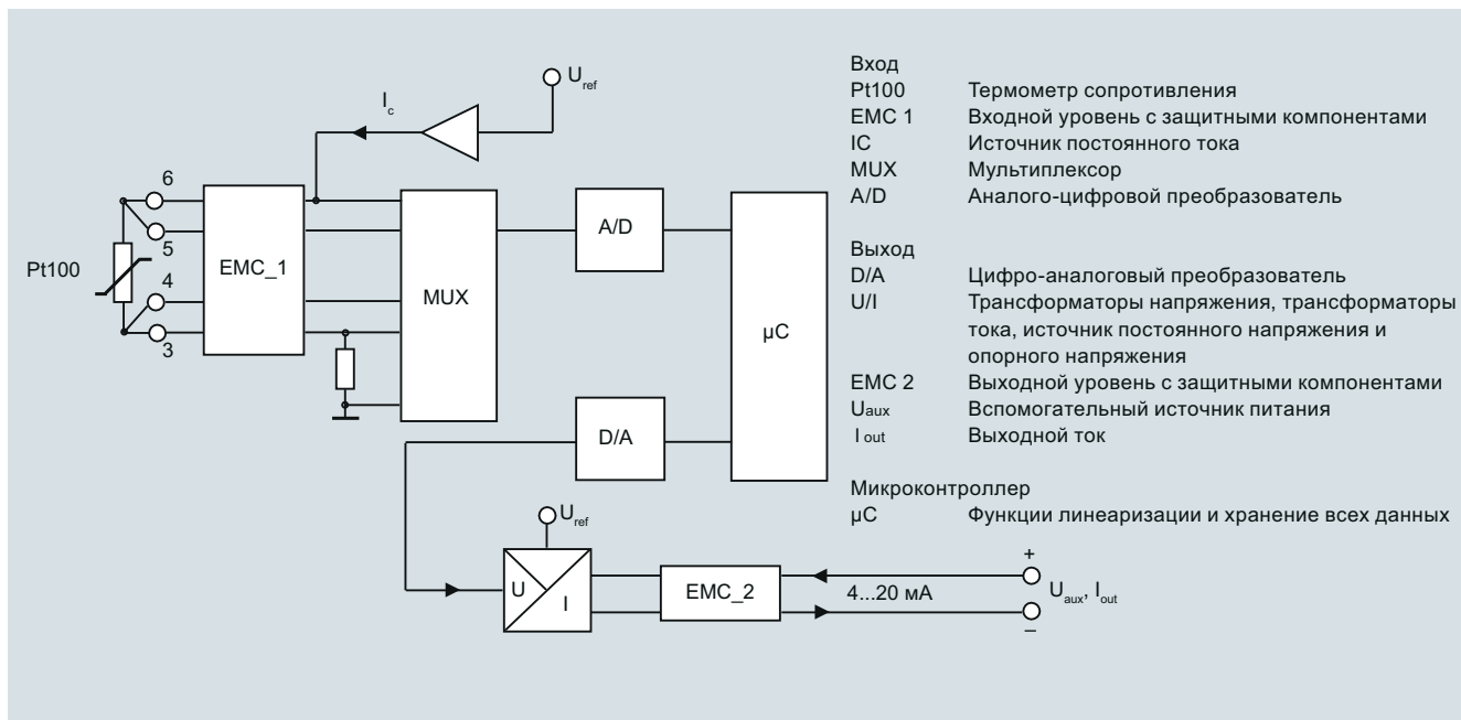
SITRANS TH100 Slim, функциональная блок-схема
