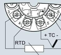
Компенсация холодного спая с внешним Pt100 в двухпроводной системе 1)
