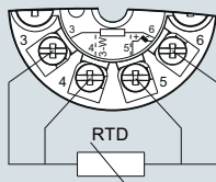
Четырехпроводная система
