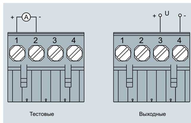
SITRANS TR320, назначение соединений выхода
