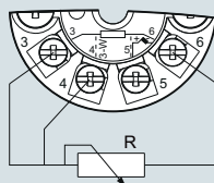
Трехпроводная система
