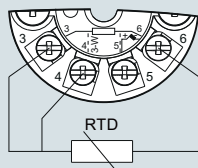
Трехпроводная система
