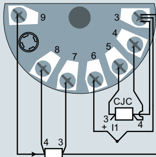
Вход 1: термопара (внутренняя КХС или внешняя 2- или 3-проводная КХС) Вход 2: 2-, 3- или 4-проводной RTD
