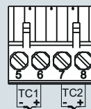
Формирование среднего значения / разности с внутренней компенсацией холодного спая
