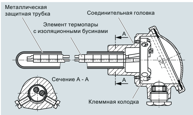
Прямая термопара с элементом из неблагородного металла Ni Cr/Ni и металлической защитной трубкой
