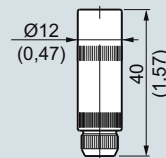
Соединитель LEMO 1S, IP50, размеры в мм (дюймах)
