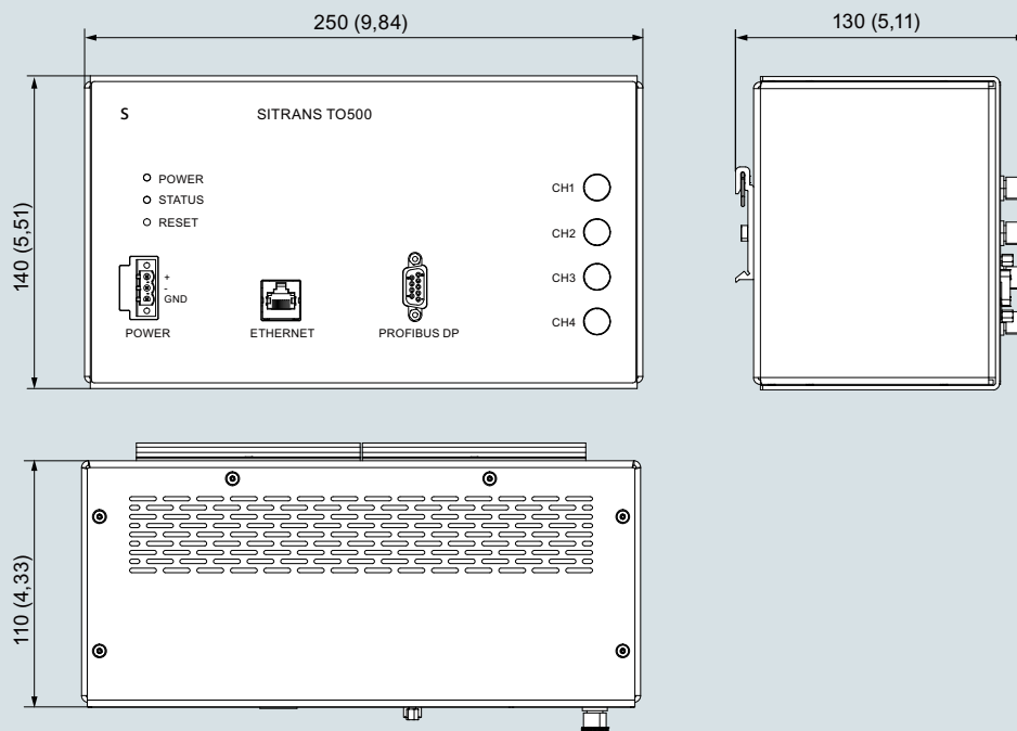
SITRANS TO500, вид спереди, сзади и сбоку; размеры в мм (дюймах)
