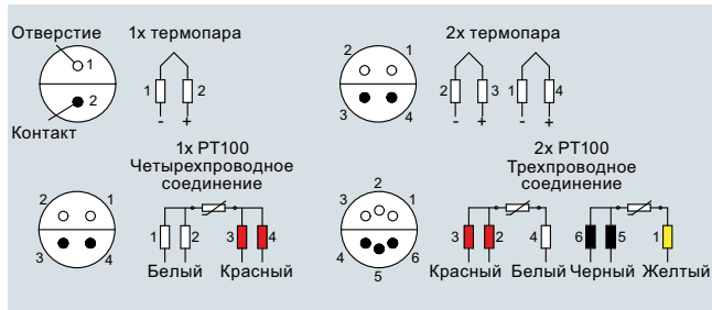
Термометр сопротивления
