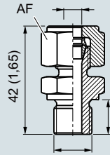
Компрессионный фитинг, метрический (A30, A31), размеры в мм (дюймах)
