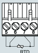
Четырехпроводная система
