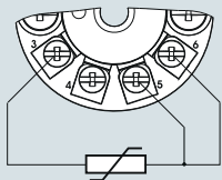
Трехпроводная система
