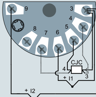
Вход 1 и/или вход 2: термопара (внутренняя КХС или внешняя 2-, 3- или 4-проводная КХС)
