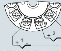
Формирование усредненного/дифференциального значения или резервирование с внутренней компенсацией холодного спая
