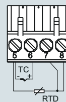
Компенсация холодного спая с внешним Pt100 в трехпроводной системе
