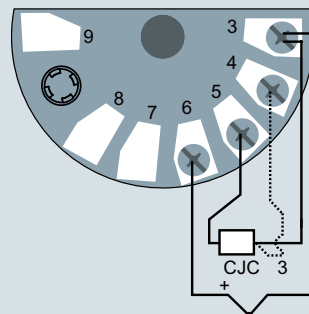
Термопара (внутренняя КХС или внешняя 2- или 3-проводная КХС)
