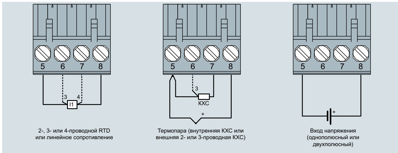
SITRANS TR320, назначение соединений входа
