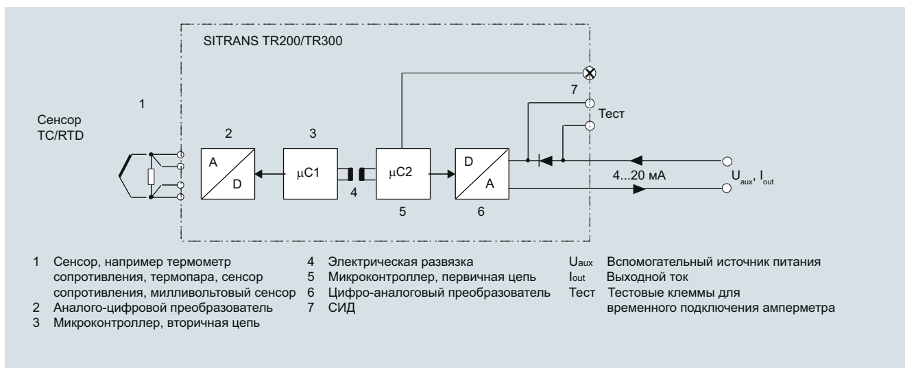
SITRANS TR200, функциональная схема
