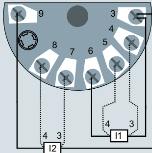
Вход 1 и/или вход 2: 2-, 3- или 4-проводной RTD или линейное сопротивление
