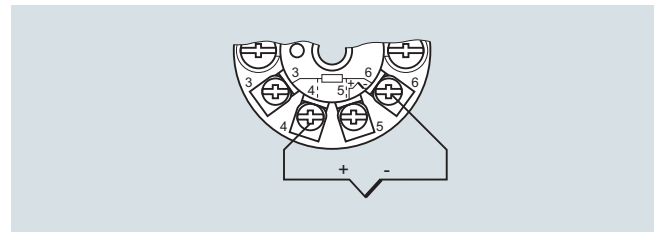
Термопары
