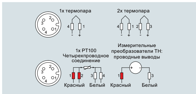
Термопары
