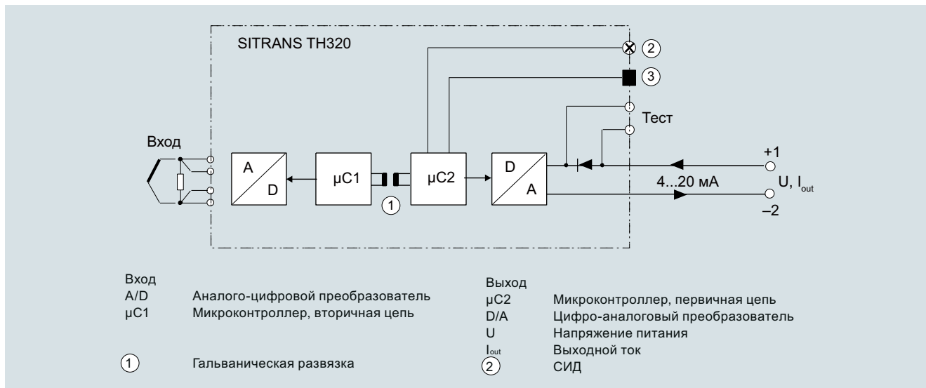
Функциональная блок-схема SITRANS TH320
