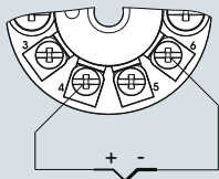
Внутренняя компенсация холодного спая
