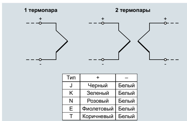
Принципиальная схема для термопары
