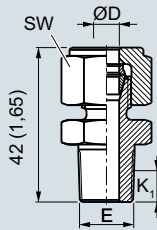
Компрессионный фитинг, NPT (A32), размеры в мм (дюймах)
