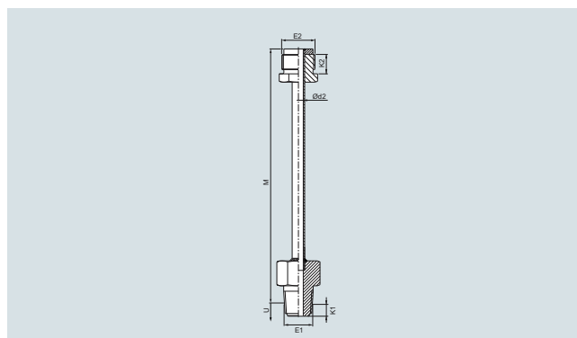
Удлинение NPT (1, 2, 3), регулируемое, европейское, коническое, размеры в мм (дюймах)
