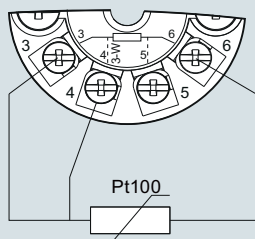
Трехпроводная система
