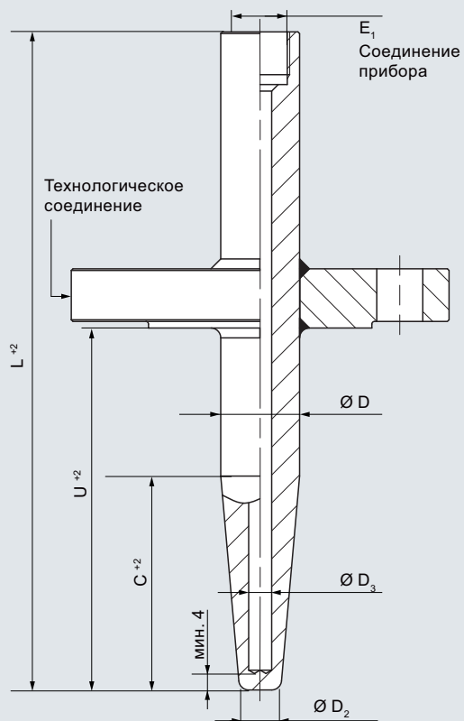
7MT14, фланцевое соединение
