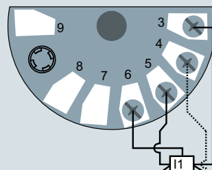
3- или 4-проводной потенциометр
