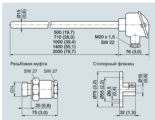
Термометр сопротивления для дымовых газов с соединительной головкой, размеры в мм (дюймах)
