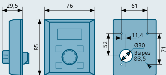
Схема сверления
