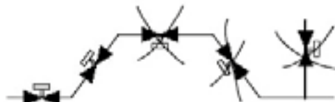
Схема расположения клапанов ДУ65-200 на трубопроводе.
