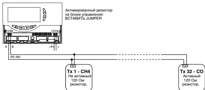
Рис. 3. Пример соединения: Блок контроля–Сенсор
