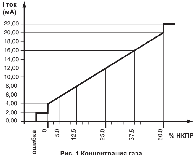
Рис. 1 Концентрация газа
