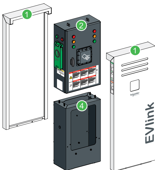
Зарядная станция для напольного монтажа
