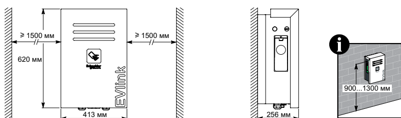
Зарядная станция для настенного монтажа
