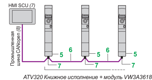
Пример подключения к машинной шине CANopen через разъем SUB-D
