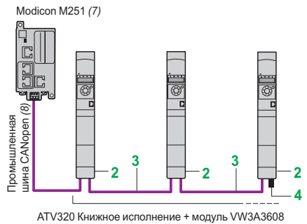
Оптимальное решение для соединения daisy chain - промышленная шина CANopen
