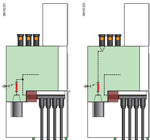
Схема подключения трансформатора напряжения для измерений на фидере
