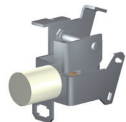
Модуль -Q0-F14 (расцепитель прямого действия)
