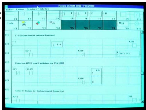
Sepam 2000
