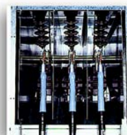
Кабельный отсек
