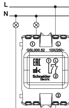
2-клавишный ВЫКЛЮЧАТЕЛЬ
