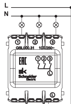
3-клавишный ВЫКЛЮЧАТЕЛЬ
