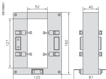
№ по кат. 16545 - 16547
