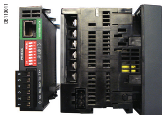
PowerLogic PM870 с модулем ECC, вид снизу (видны разъемы и переключатели конфигурации)
