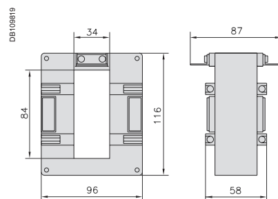
№ по кат. 16537 и 16538
