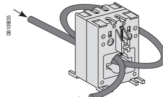
Эквивалентен ТТ 100/5 А, I_{\text{макс.}} = 50 \text{ А}
