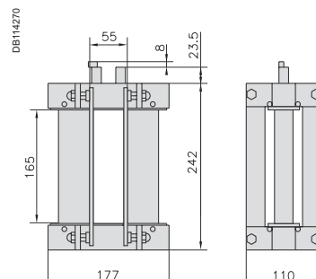
№ по кат. 16548 - 16549
