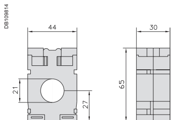
№ по кат. 16500, 16451 - 16456
