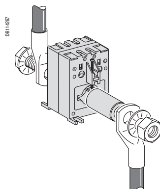
ТТ с присоединением кабеля с помощью винта и гайки Применяются втулки 16550 или 16551
