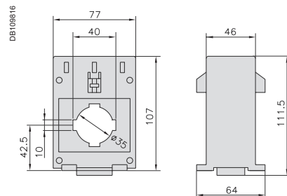
№ по кат. 16468 - 16471
