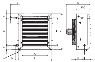
Ø 1/2" Слив конденсат
