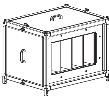
Карманный фильтр
