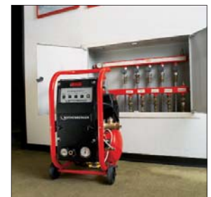
Промывка системы отопления пола
