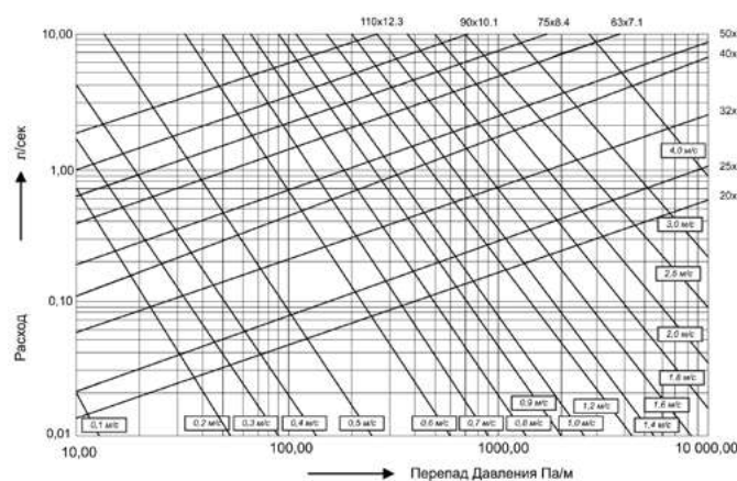
Номограмма потерь давления для труб РОСТерм FRP, армированных стекловолокном, SDR7,4/SDR9 при температуре 90 °С
