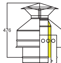
Дефлектор конический
