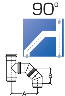
2 отвода 45°, 1 тройник 90°
