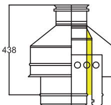
Окончание коническое-переход
