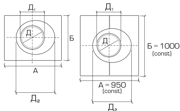
Основа нержавеющая
