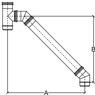
2 отвода 45°, 1 труба 1000, 1 тройник 90°
