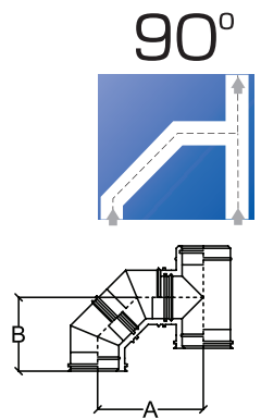
2 отвода 45°, 1 тройник 90°
