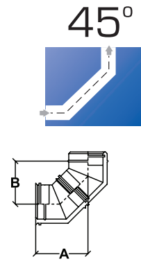
2 отвода 45°
