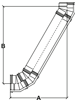
2 отвода 30°, 1 труба 1000
