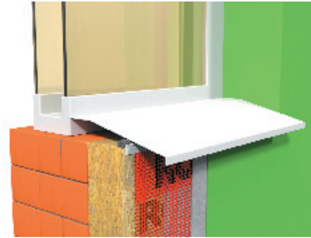
Рисунок 9. Профиль примыкающий угловой с сеткой и ПСУЛ
