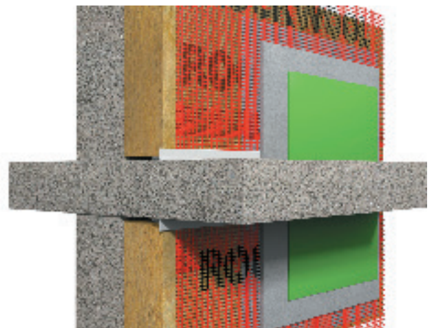
Рисунок 8. Профиль примыкающий угловой с сеткой и ПСУЛ
