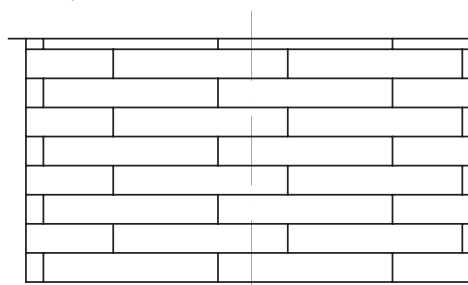
Схемы установки дюбелей Краевая зона Рядовая зона
