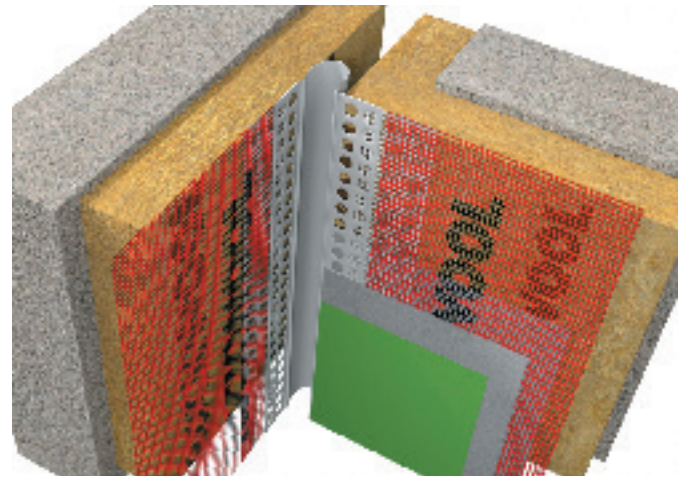
Рисунок 12. Профиль деформационный угловой
