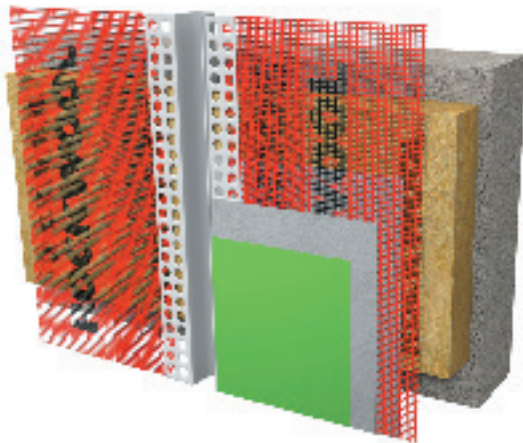
Рисунок 13. Профиль деформационный плоскостной
