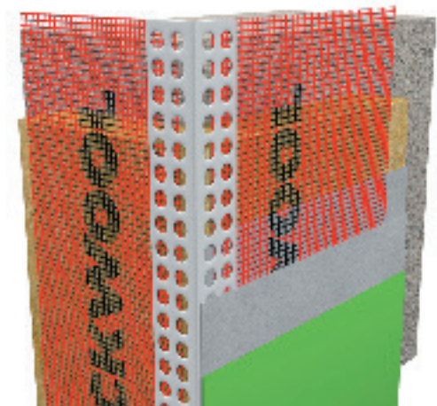
Рисунок 2. Профиль угловой армирующий
