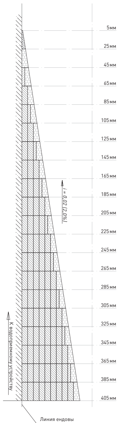
Продольный разрез Конструктивов (КУ 600; КУ 300; КУ 200) с длиной элементов 1000 мм системы ROCKWOOL РУФ УКЛОНА
