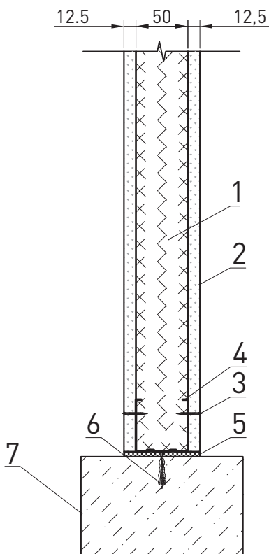
Перегородка 75 мм АКУСТИК БАТТС 50 мм 1 слой гипсокартона
