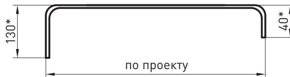
КОСТЫЛЬ К4
