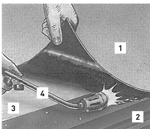
Рисунок 6. Наклейка основного водоизоляционного ковра на карнизе
