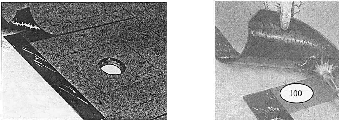
Рисунок 4. Сопряжение (нахлестка) изоляционных слоев на примыкании к воронке внутреннего водостока
