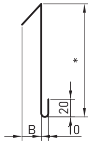
НАЩЕЛЬНИК Н1
