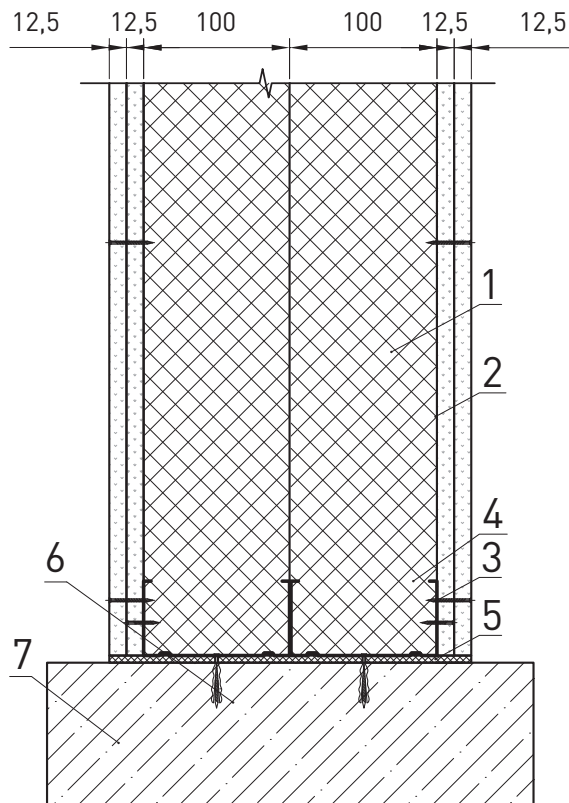
Перегородка 250 мм АКУСТИК БАТТС 200 мм 2 слоя гипсокартона
