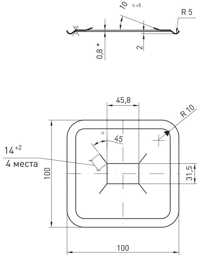
ПРИЖИМНАЯ ПЛАНКА
