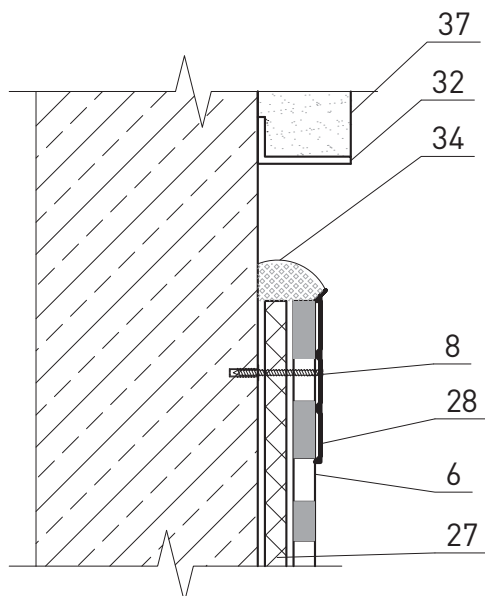
Узел 2.1-3
