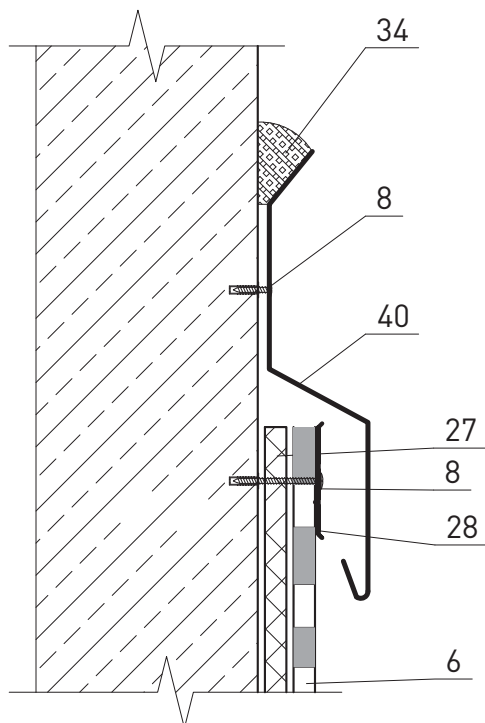
Узел 2.1-3
