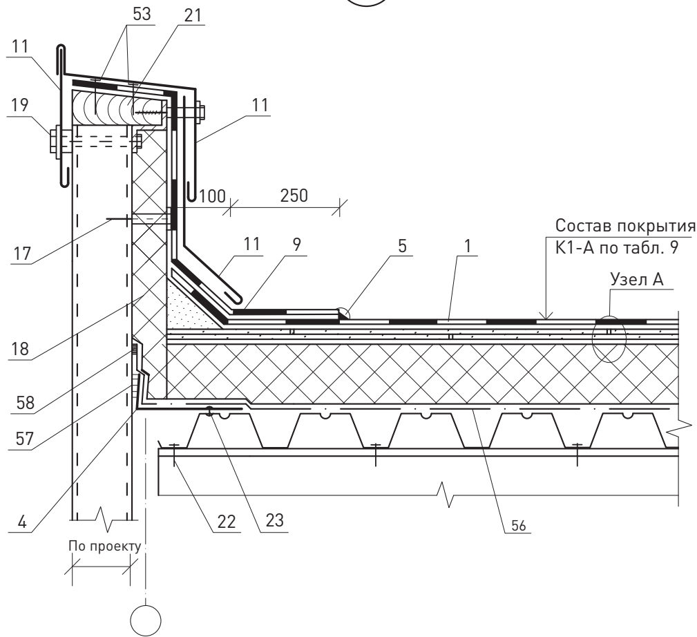
Узел А
