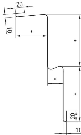
НАЩЕЛЬНИК Н5
