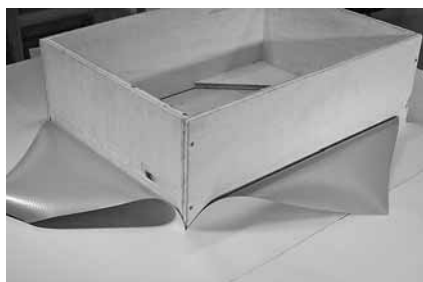
Рисунок 1.1. При устройстве примыкания кровельной мембраны к вертикальным поверхностям на внешних углах вентиля и т.п. (световой фонарь, парапет и др.) мембрану разрезают под углом 45°.
