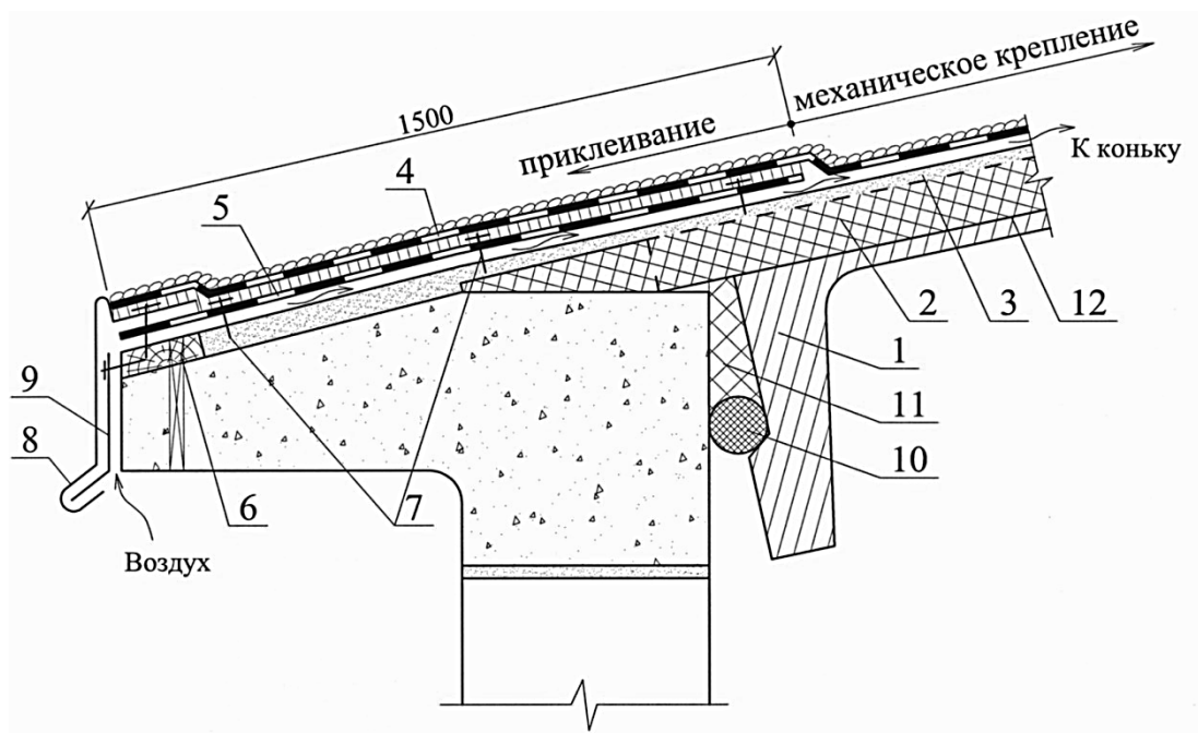
Рисунок 7. Водоизоляционный ковер на карнизе
