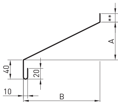
СЛИВ С1
