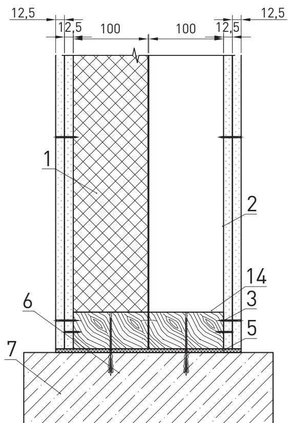
Перегородка 250 мм АКУСТИК БАТТС 100 мм 2 слоя гипсокартона
