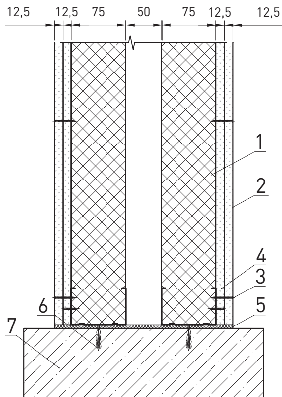
Перегородка 250 мм АКУСТИК БАТТС 150 мм 2 слоя гипсокартона
