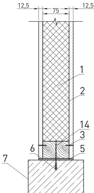
Перегородка 100 мм АКУСТИК БАТТС 75 мм 1 слой гипсокартона
