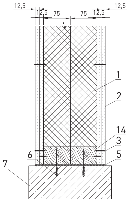
Перегородка 200 мм АКУСТИК БАТТС 150 мм 2 слоя гипсокартона
