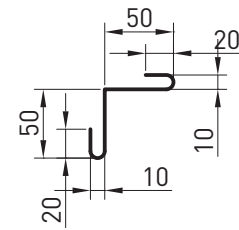
НАЩЕЛЬНИК Н4
