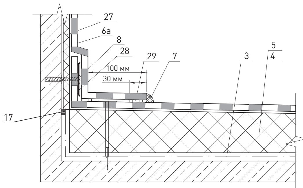
Узел 1.2-3
