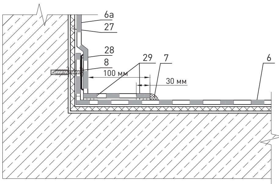
Узел 1.2-1
