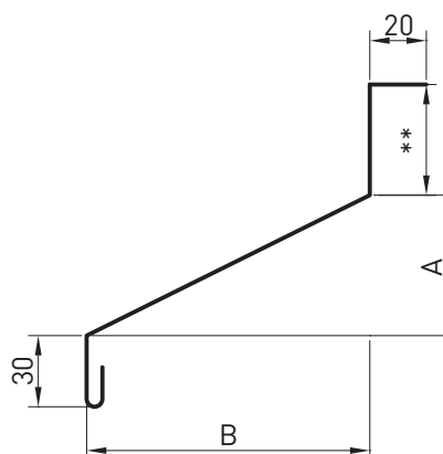
СЛИВ С5
