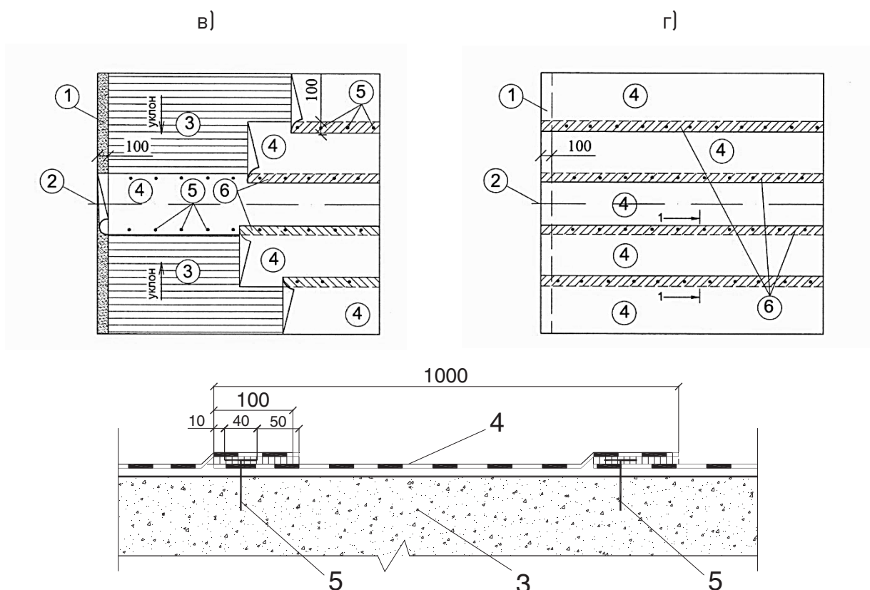
Рисунок 2. Раскладка нижнего слоя водоизоляционного ковра из рулонного битумно-полимерного материала с механическим закреплением
