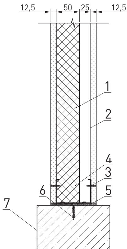
Перегородка 100 мм АКУСТИК БАТТС 50 мм 1 слой гипсокартона
