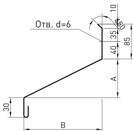
СЛИВ С3
