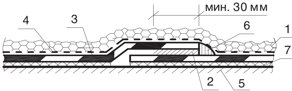
Рисунок 11. Стык смежных полотнищ пленки с пригрузом
