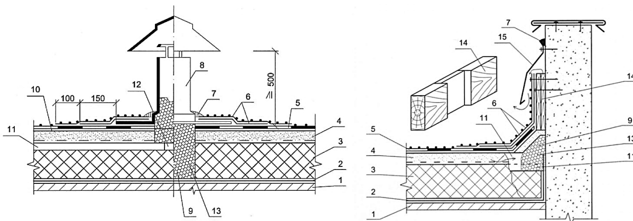
Рисунок 10. Осушающий патрубок (а) и примыкание каналов к стене с продухом (б)
