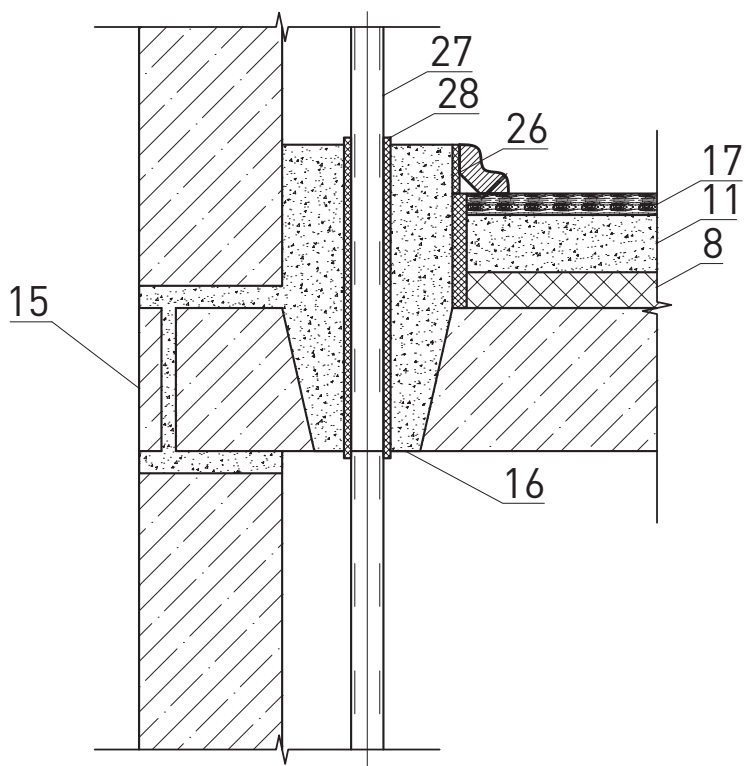
Звукоизоляция трубопроводов при их проходке через межэтажное перекрытие
