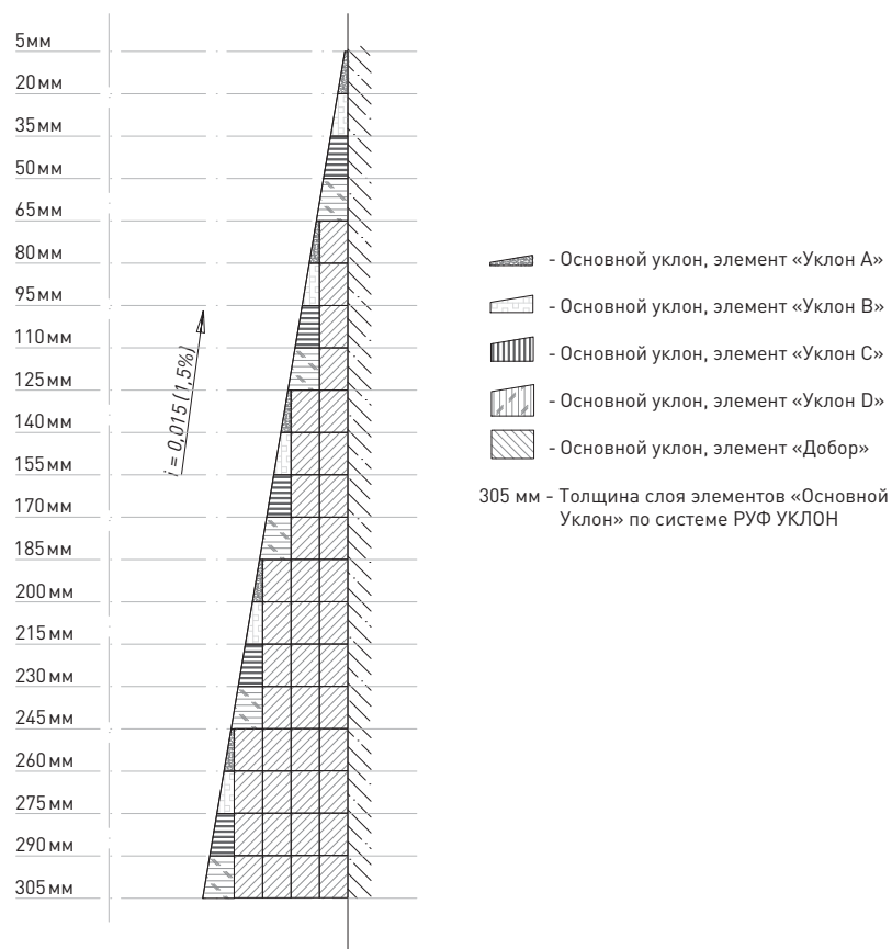
Геометрические размеры элементов набора «Основной уклон»
