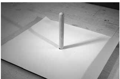
Рисунок 4.1. Для герметизации такого элемента в кровле (громоотводы, абели, стойки крепления и другие) вырезают из неармированной мембраны круг радиусом около 150 мм.
