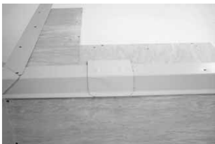
Рисунок 5.3. Стык между профилями из ламинированной ПВХ-жести заваривают полосой неармированной ПВХ-мембраны ROCKmembrane шириной около 20 см.
