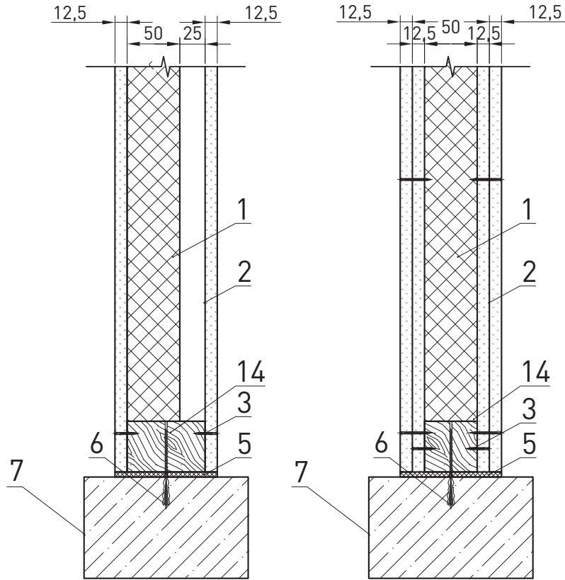
Перегородка 100 мм АКУСТИК БАТТС 50 мм 1 слой гипсокартона
