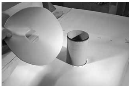
Рисунок 3.1. Для герметизации примыкания кровельной мембраны к трубе надо вырезать кольцо из неармированной мембраны с внешним диаметром на 200 мм больше диаметра трубы и внутренним диаметром на 50 мм меньше диаметра трубы.
