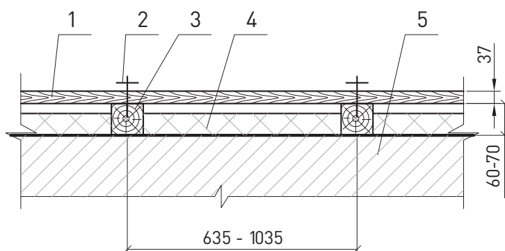
Полы с дощатым покрытием на лагах и звукоизоляцией из плит АКУСТИК БАТТС или АКУСТИК БАТТС ПРО
