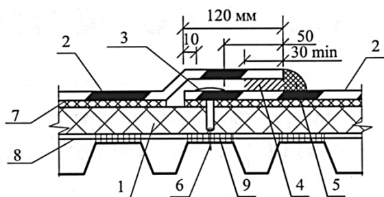
Рисунок 16. Стык смежных полотнищ рулонного материала
