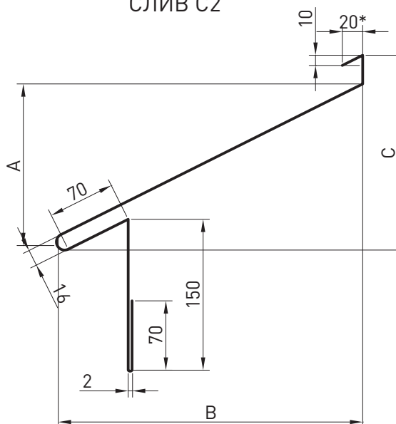
СЛИВ С2
