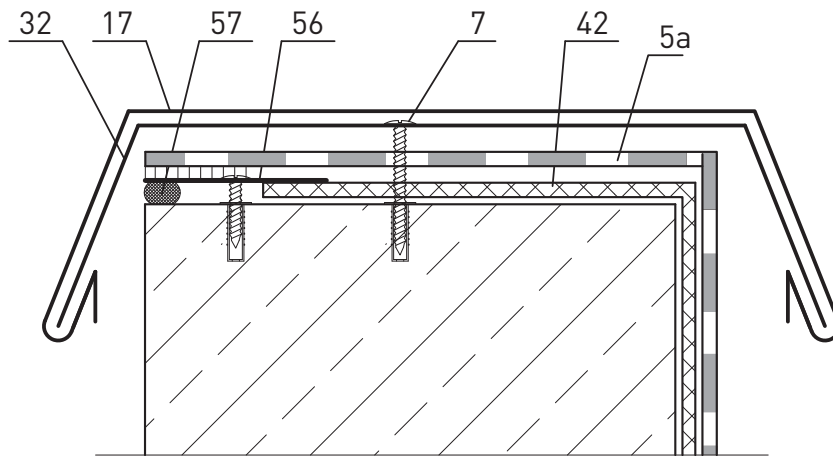
Узел 1.1
