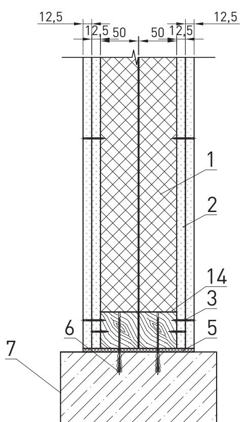
Перегородка 150 мм АКУСТИК БАТТС 100 мм 2 слоя гипсокартона
