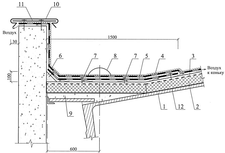
Рисунок 9. Примыкание водоизоляционного слоя к парапету
