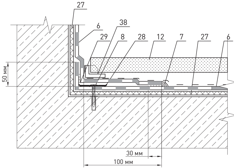
Узел 2.2-2
