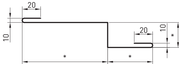
НАЩЕЛЬНИК Н3
