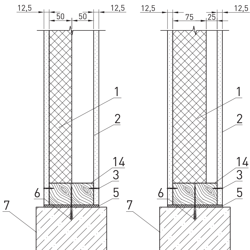
Перегородка 125 мм АКУСТИК БАТТС 50 мм 1 слой гипсокартона
