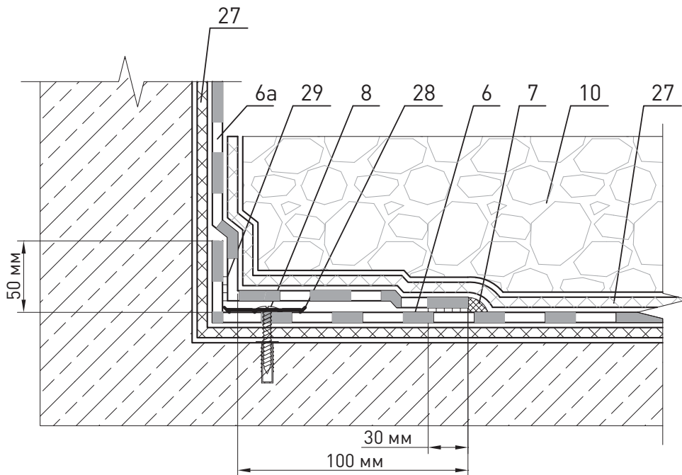
Узел 2.2-2
