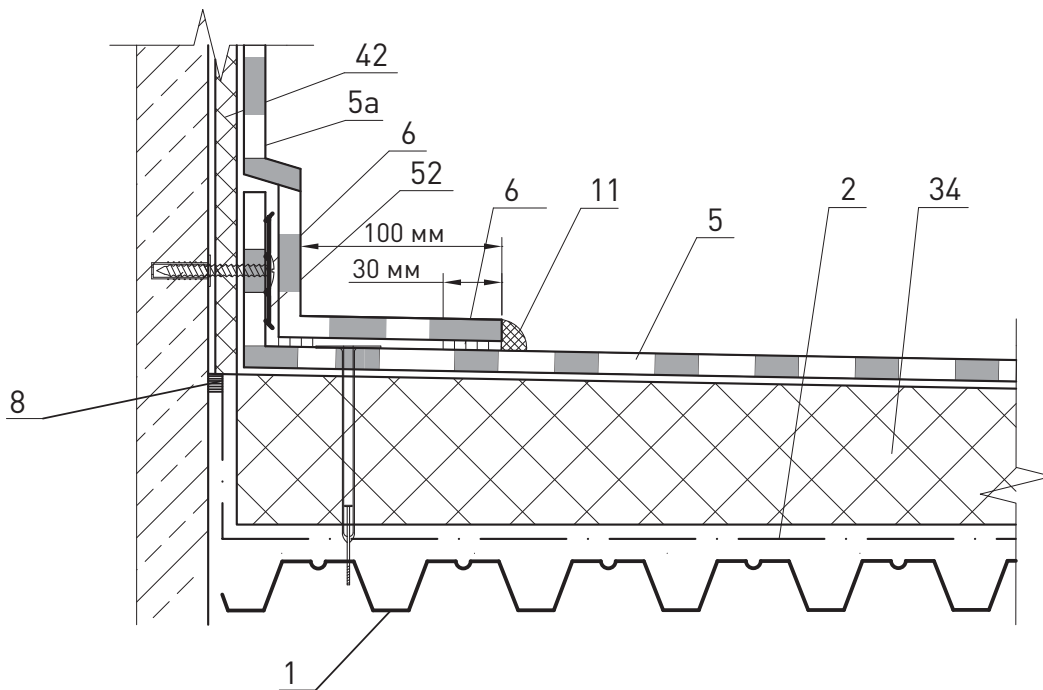
Узел 1.2 - 3
