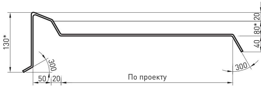
КОСТЫЛЬ К3
