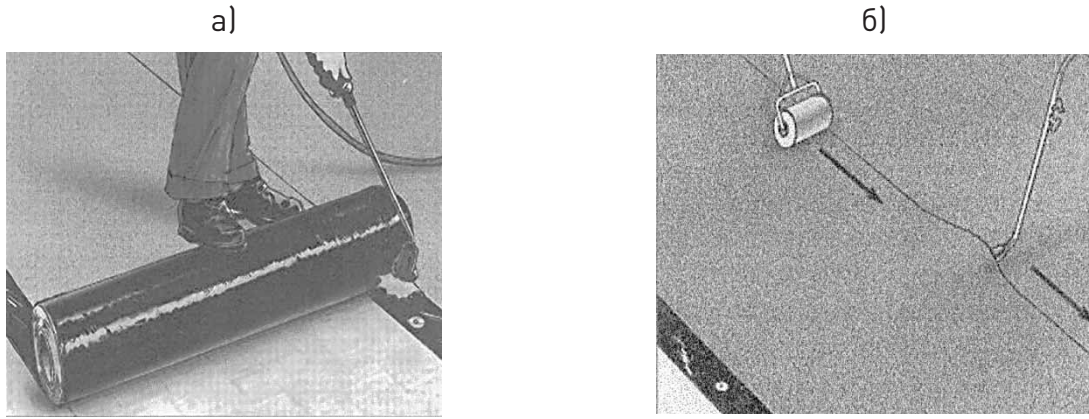
Рисунок 1. Разогрев кромок рулонного материала в местах нахлестки пламенем газовой горелки (а) и с прикаткой роликом шириной 100 мм (б)
