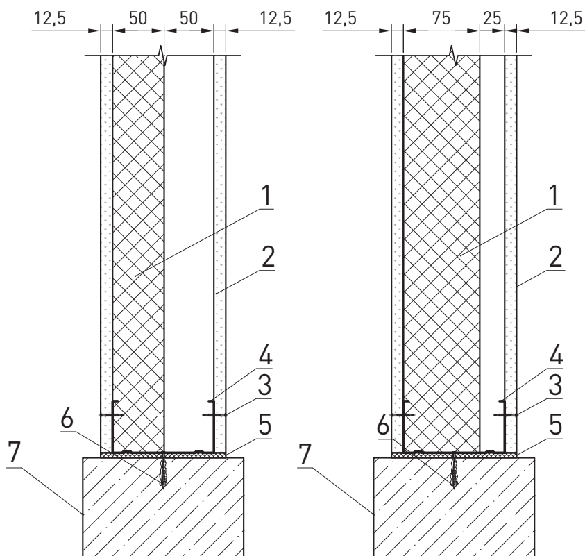
Перегородка 125 мм АКУСТИК БАТТС 50 мм 1 слой гипсокартона
