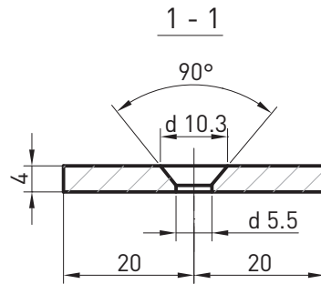
КОСТЫЛЬ К3
