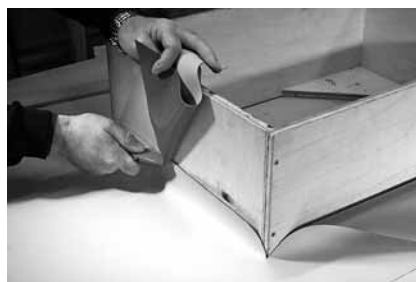
Рисунок 1.2. Мембрану заводят с горизонтальной на вертикальную или наклонную поверхность на высоту около 50 мм.
