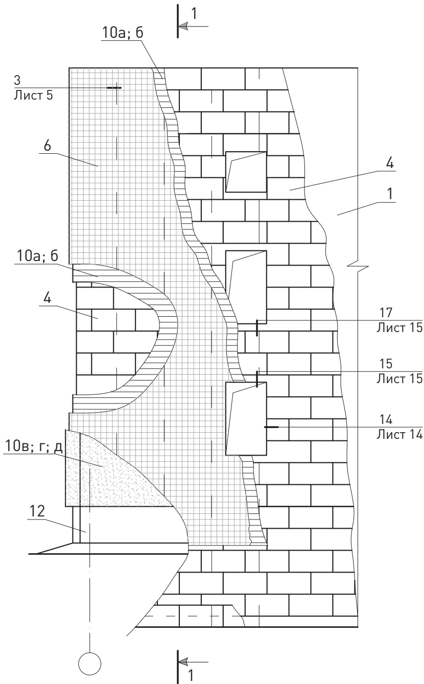
СХЕМА № 1. Расположение плит утеплителя, сетки и штукатурки
