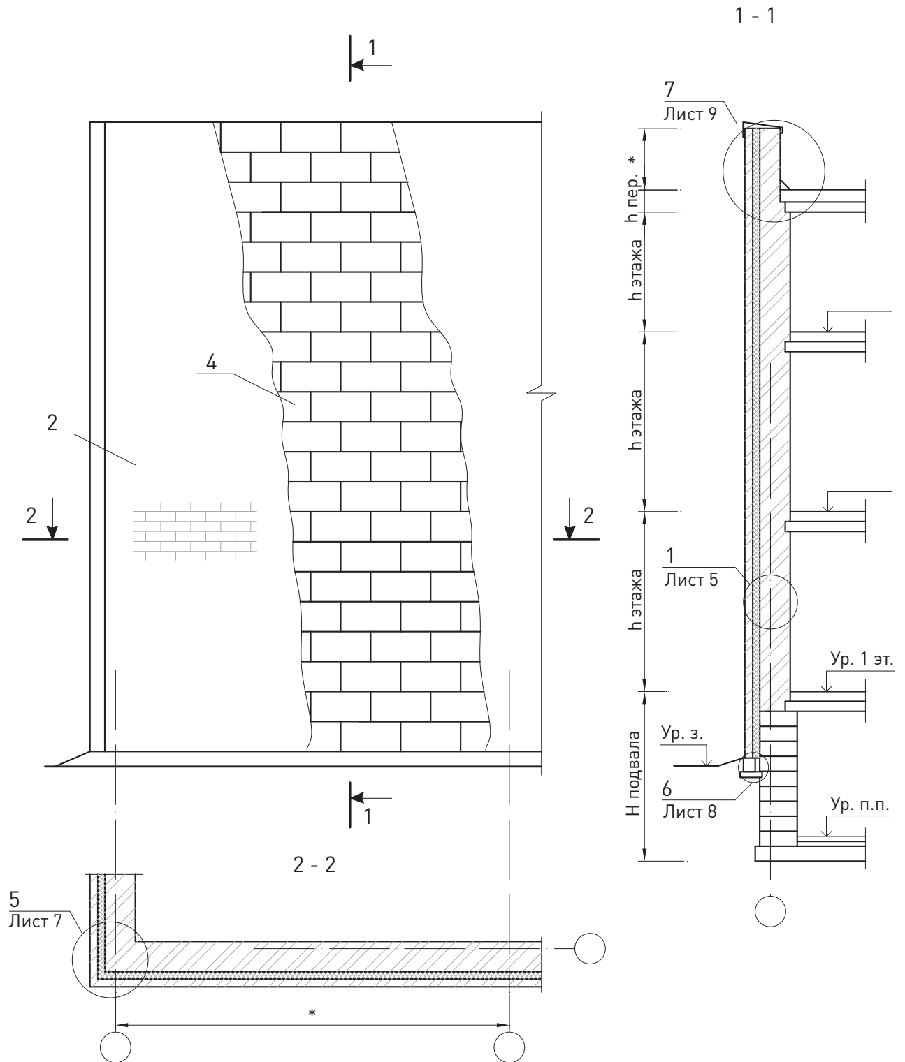
СХЕМА № 1. Расположение плит утеплителя, расщечек
