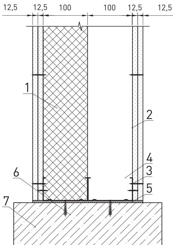
Перегородка 250 мм АКУСТИК БАТТС 100 мм 2 слоя гипсокартона
