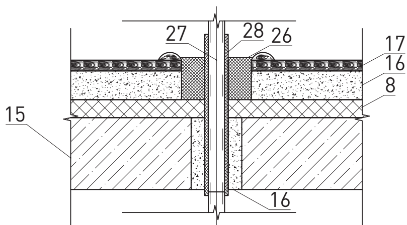
Звукоизоляция трубопроводов при их проходке через межэтажное перекрытие
