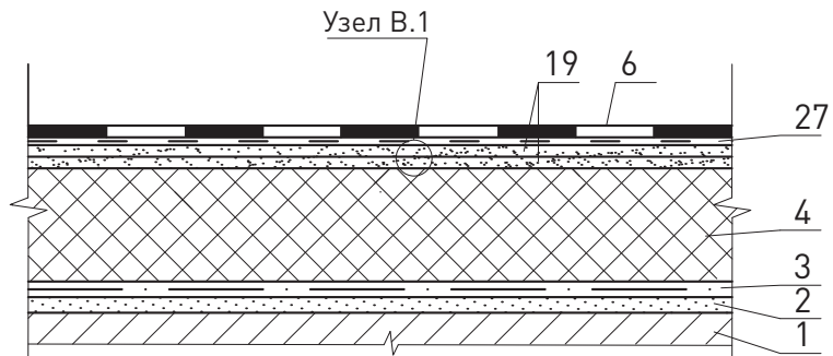
Узел "В.1"
