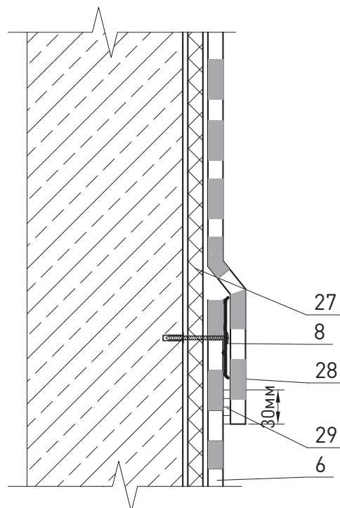
Узел 2.1-4
