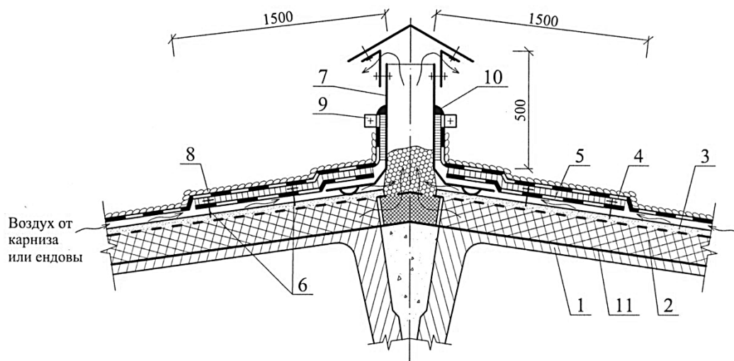
Рисунок 8. Водоизоляционный слой на коньке
