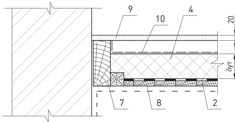
Чердачное перекрытие с деревянными несущими балками
