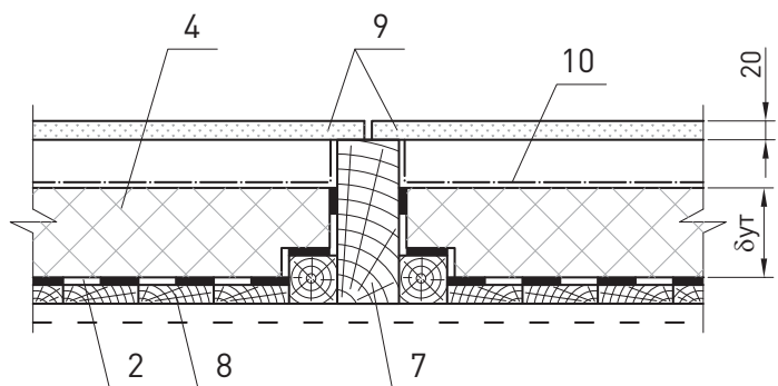
По средней несущей балке 1 - 1
