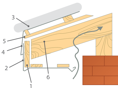
Рис. 7.5. Устройство продухов в подшивке карниза: 1 — карнизная доска; 2 — карнизная подшивочная планка; 3 — кровельное покрытие; 4 — карнизная планка; 5 — контрообрешетка; 6 — стропильная нога.
