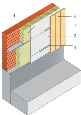
Рис. 1.8. Устройство вентилируемой воздушной прослойки в стенах с обшивкой сайдингом: 1 — плиты ROCKWOOL ЛАЙТ БАТТС® или Лайт Баттс СКАНДИК; 2 — мембрана ROCKWOOL для стен; 3 — вентилируемая воздушная прослойка; 4 — внутренняя стена; 5 — наружная обшивка.
