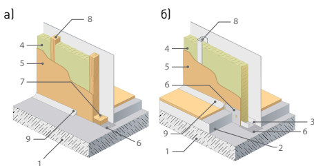
Рис. 2.1. Каркасно-обшивные перегородки с деревянным (а) и металлическим каркасом (б):
