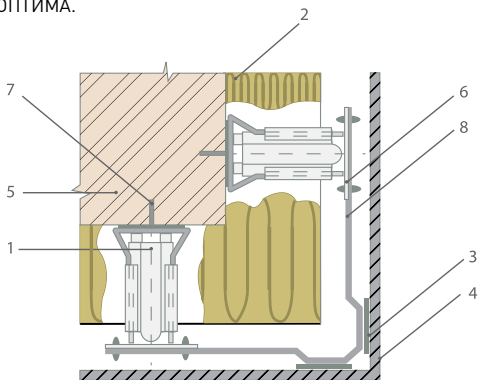
Рис. 1.27. Схема крепления облицовки и плит ROCKWOOL ВЕНТИ БАТТС® в зоне наружного угла здания:
