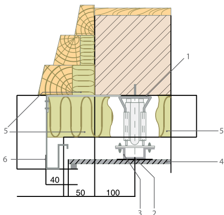
Рис. 1.26. Узел примыкания навесной фасадной системы к оконному проему:
