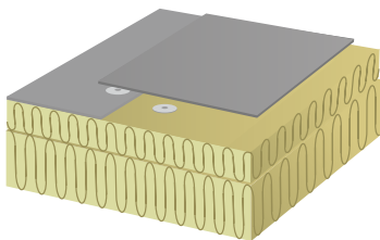
Рис. 7.15. Крепление гидроизоляционной мембраны к покрытию
