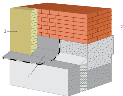
Рис. 1.11. Устройство гидроизоляционного слоя: 1 — гидроизоляция; 2 — утепляемая стена; 3 — плиты ROCKWOOL КАВИТИ БАТТС®.
