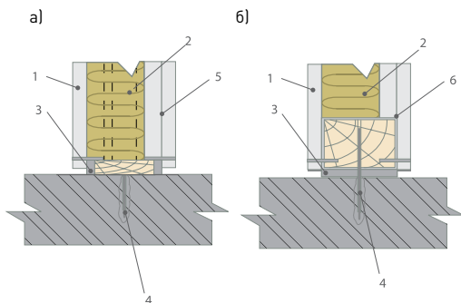
Рис. 2.3. Опираие перегородок на междуэтажное перекрытие:
