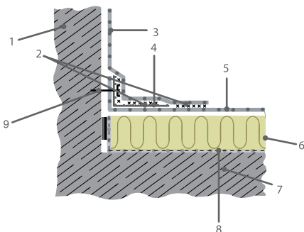
Рис. 7.17. Примыкание системы ROCKROOF к вертикальной стене и водосточной воронке
