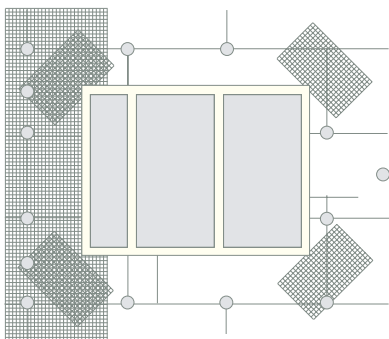
Рис. 1.21. Раскладка утеплителя с перевязкой швов, устройство технологических вырезов в плитах утеплителя около проемов, установка дополнительных косынок из стеклотетки.
