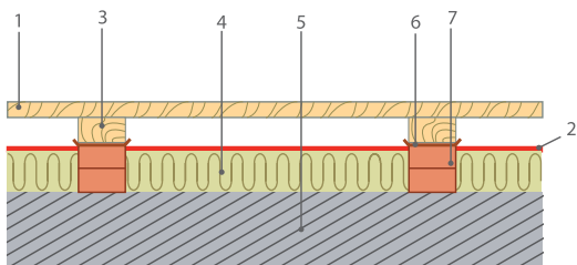
Рис. 4.5. Утепление плитного перекрытия с лагами по столбикам: 1 — покрытие пола ; 2 — пароизоляция ROCKWOOL; 3 — лага; 4 — плиты ROCKWOOL ЛАЙТ БАТТС® или Лайт Баттс СКАНДИК требуемой толщины; 5 — плита перекрытия; 6 — прокладки из рубероида; 7 — столбик из кирпича или брусек из легкого бетона.
