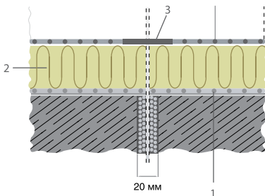
Рис. 7.16. Изоляция деформационного шва 1 — пароизоляция ROCKbarrier, 2 — теплоизоляция ROCKWOOL, 3 — дополнительный слой.
