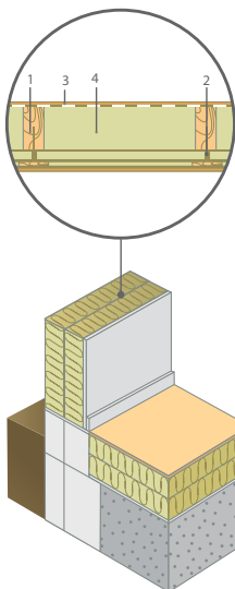
Рис. 1.6. Каркасно-обшивная стена с брусками, прикрепленными к стойкам каркаса:
