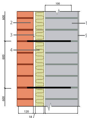
Рис. 1.16. Трехслойная кирпичная стена с утеплением плитами ROCKWOOL КАВИТИ БАТТС®:
