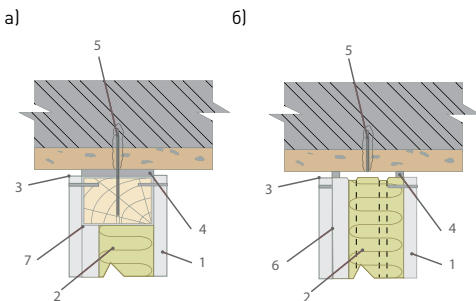
Рис. 2.2. Примыкание перегородок к верхнему перекрытию:
