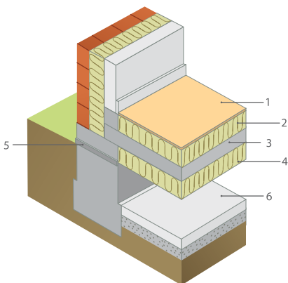
Рис. 4.6. Дополнительное утепление перекрытия над подвалом: 1 — покрытие пола; 2 — плиты ROCKWOOL ФЛОР БАТТС®; 3 — плита перекрытия; 4 — дополнительное утепление плитами ROCKWOOL ВЕНТИ БАТТС®; 5 — вентиляционный продух; 6 — пол холодного подвала.
