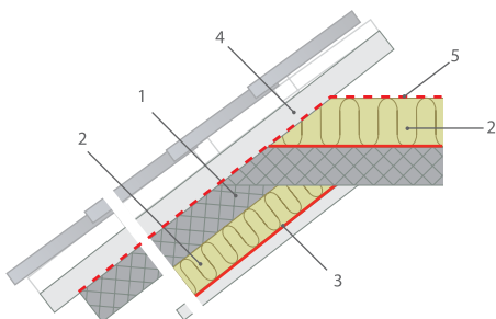
Рис. 7.7. Дополнительное утепление мансарды:
