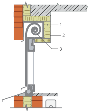
Рис. 1.14. Утепление полости для свернутых роль-ставней: 1 — плиты ROCKWOOL ЛАЙТ БАТТС® или Лайт Баттс СКАНДИК; 2 — внутренняя отделка утепляющего короба; 3 — роль-ставни.
