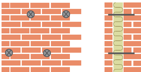
Рис. 1.13. Установка связей между внутренней и наружной стенками в трехслойной стене.
