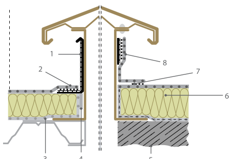
Рис. 7.13. Примыкание пароизоляции ROCKbarrier и гидроизоляционной мембраны ROCKmembrane к выступающим элементам на покрытии. 1 — ламинированная ПВХ жёсть; 2 — ПВХ мембрана; 3 — пароизоляция; 4 — склеивающая лента; 5 — перекрытие; 6 — плиты ROCKWOOL РУФ БАТТС®, ROCKWOOL РУФ БАТТС ОПТИМА®, ROCKWOOL РУФ БАТТС ЭКСТРА®; 7 — герметик; 8 — ламинированная ПВХ жёсть.
