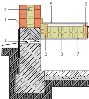
Рис. 4.1. Устройство продухов для вентиляции подполья:
