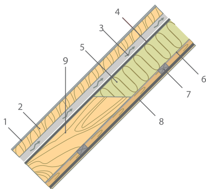
Рис. 7.3. Покрытие мансарды:
