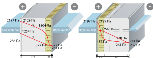
Рис. 1.3. Характер распределения упругости водяных паров в кирпичной стене толщиной 510 мм, утепленной плитами из каменной ваты толщиной 120 мм, при температуре внутреннего воздуха t_{в} = 20^{\circ}\text{C} , его относительной влажности j_{в} = 55\% и температуре наружного воздуха t_{н} = -28^{\circ}\text{C} и его относительной влажности 83%.
