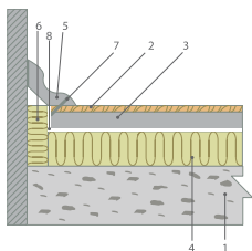
Рис. 3.3. Примыкание полов к стенам и перегородкам:
