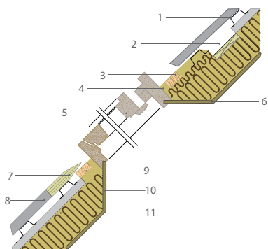
Рис. 7.8. Установка оконных блоков для освещения мансардных помещений:
