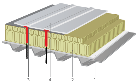
Рис. 7.12. Компоненты системы ROCKROOF:
