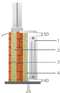
Рис. 1.15. Установка отопительного прибора:
