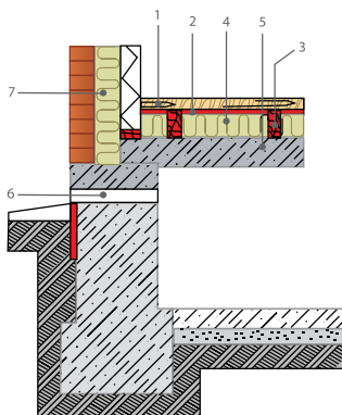
Рис 4.4. Утепление плитного перекрытия над холодным подвалом
