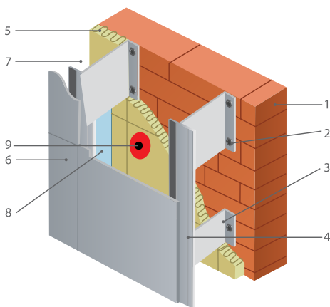
Рис. 1.25. Конструкция навесного фасада с воздушным зазором: 1 — утепляемая стена; 2 — распорный анкер; 3 — кронштейн; 4 — направляющие; 5 — плиты серии ВЕНТИ БАТТС®; 6 — плиты защитной декоративной облицовки (например, ROCKPANEL); 7 — воздушный зазор; 8 — вставка кронштейна; 9 — фасадный дюбель.
