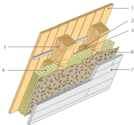
Рис. 7.2. Покрытие мансарды:
