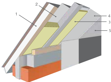
Рис. 7.1. Покрытие мансарды:
