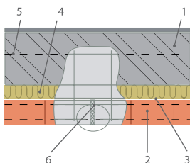
Рис. 1.18. Деформационные швы в слоистой кладке: 1 — внутренняя часть стены; 2 — наружная защитно-декоративная кладка толщиной 120 мм; 3 — воздушный зазор; 4 — плиты ROCKWOOL КАВИТИ БАТТС®; 5 — армирующая сетка; 6 — мастика.
