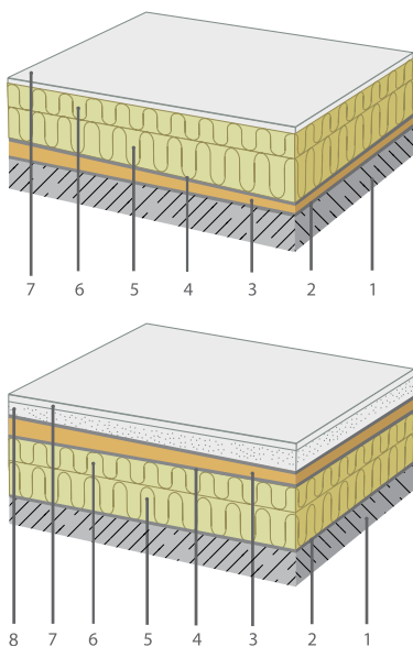
Рис. 7.10. Устройство уклона плоского покрытия при основании плоского покрытия из железобетонной плиты: 1 — плита перекрытия; 2 — пароизоляция; 3 — керамзитовый гравий, пролитый цементно-песчаным раствором; 4 — разделительный слой; 5 — плиты ROCKWOOL РУФ БАТТС Н®; 6 — плиты ROCKWOOL РУФ БАТТС В®; 7 — гидроизоляция; 8 — цементно-песчаная стяжка, армированная металлической сеткой.
