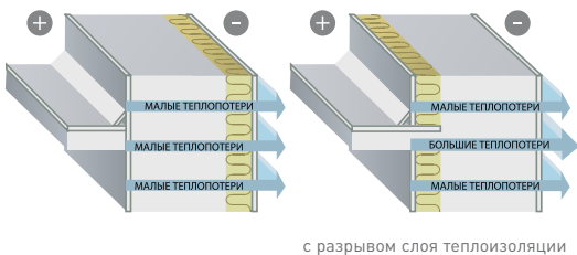
Рис. 1.4. Схема расположения утеплителя при дополнительном утеплении стен существующих зданий с наружной и внутренней стороны.
