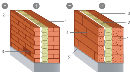
Рис. 1.9. Устройство вентиляционных продухов в кирпичной стенке:
