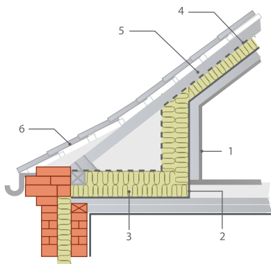
Рис. 7.6. Установка изоляционного материала по всей поверхности конструкций, граничащих с наружной средой:
