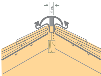
Рис. 7.4. Схема устройства коньковых продухов
