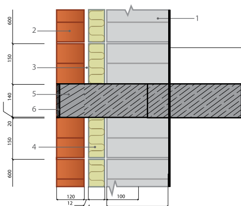
Рис. 1.19 Устройство несущих поясов в защитно-декоративной стенке: 1 — внутренняя часть стены; 2 — наружная защитно-декоративная кладка толщиной 120 мм; 3 — воздушный зазор; 4 — плиты ROCKWOOL КАВИТИ БАТТС®; 5 — несущая балка-пояс; 6 — мастика.
