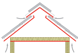
Рис. 5.4. Расположение вентиляционных продухов на чердаке.
