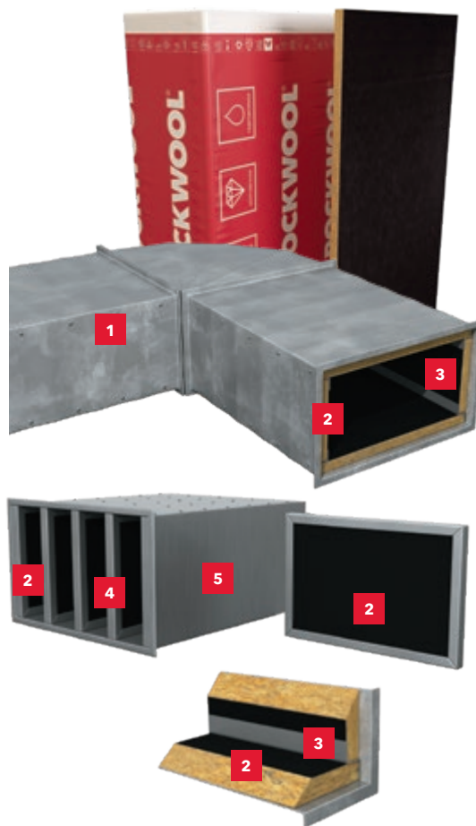
Рисунок 9. Примеры монтажа
