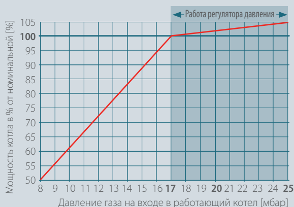
► Мощность котла и давление газа на входе (для PLATINUM)
