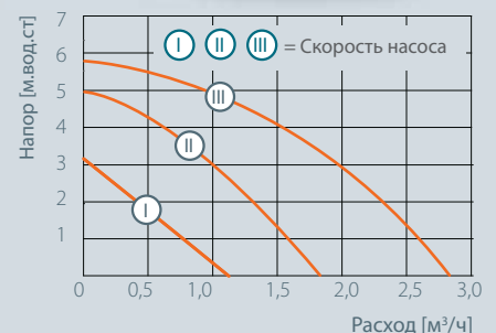
► Характеристика насоса PLATINUM
