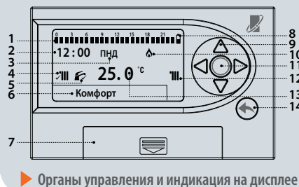
► Органы управления и индикация на дисплее
