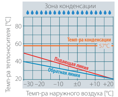
► Зона конденсации | Теплый пол 50/40°C
