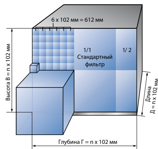
Одна шестая фильтра 1/1 = 102 мм x 102 мм
