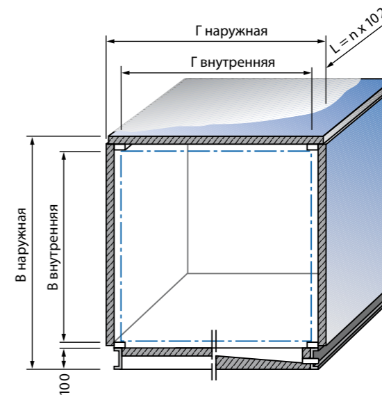
Размеры корпуса
