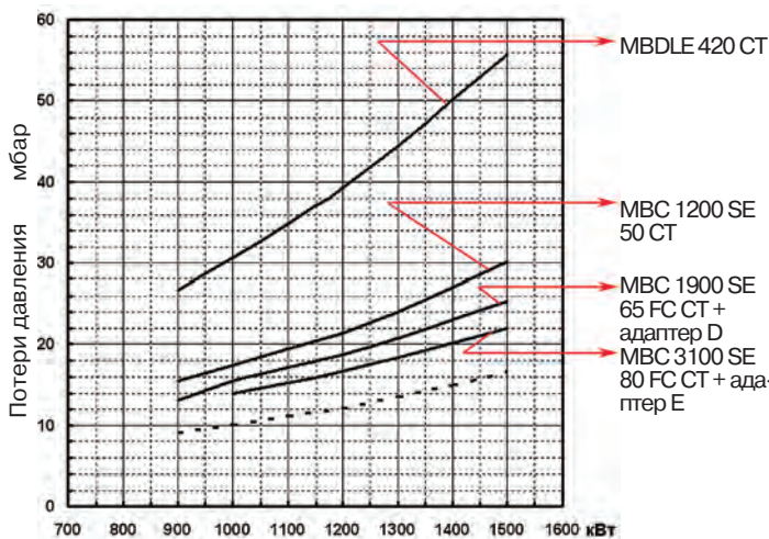
ENNE/EMME 1400 HS
