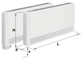
MVP-MVR+pedini * distanza da terra
