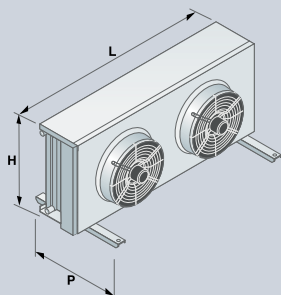
Installazione verticale (V)
