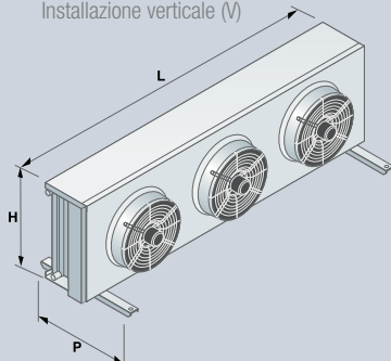
Installazione verticale (V)
