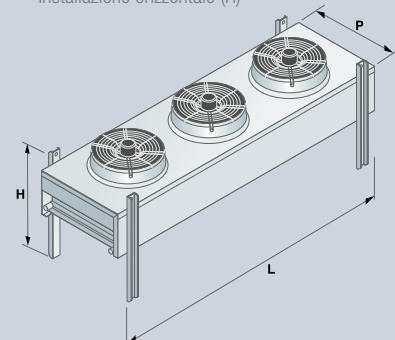
Installazione orizzontale (H)
