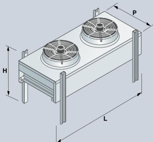
Installazione orizzontale (H)
