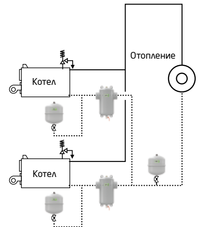
Exdirt "Сталь" - пример монтажа
