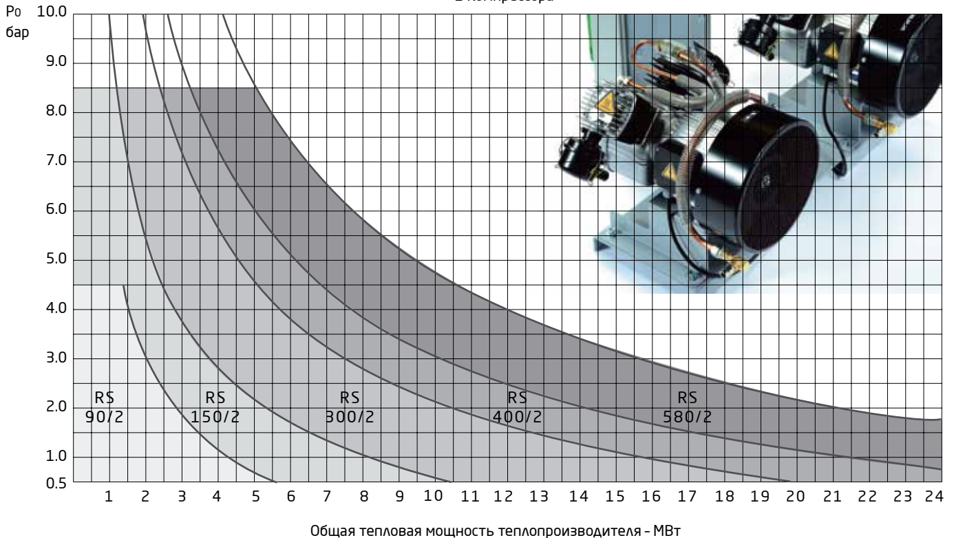
2 Компрессора
