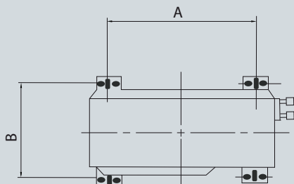
Установочные размеры
