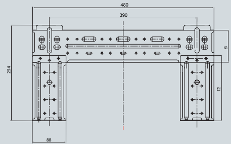
Монтажная пластина QV/QN-E12WA
