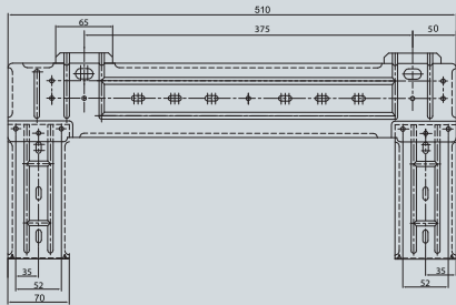
Монтажная пластина QV/QN-E09WA
