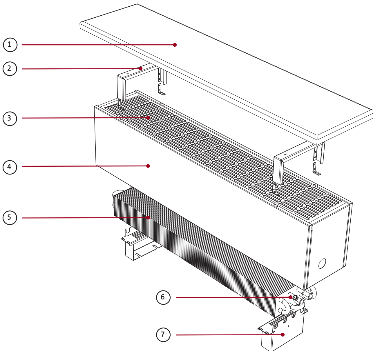
Устройство конвектора Aura Bench
