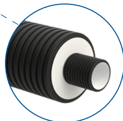
Трубы ИЗОКОРСИС (АРКТИК-УК)
