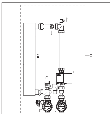
задняя плоскость, накопительный контур (вторичный контур X-Uuo 25)
