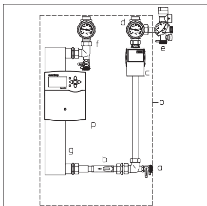
передняя плоскость, солнечный контур (первичный контур X-Uuo 25 и X-Duo 25)
