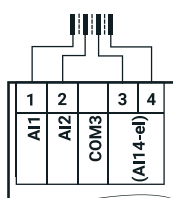
Подключение кондуктометрических датчиков: четырехпроводная схема
