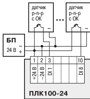
ПЛК100-24, датчик р-р-п-типа
