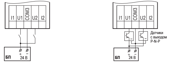
Подключение к универсальным входам, работающим в дискретном режиме, датчиков типа «сухой контакт» / Подключение к универсальным входам, работающим в дискретном режиме, трехпроводных дискретных датчиков, имеющих выходной транзистор р-п-р-типа с ОК
