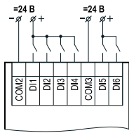
Подключение к дискретным входам типа «Д» датчиков типа «сухой контакт»
