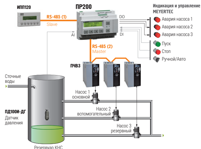
Автоматизация КНС
