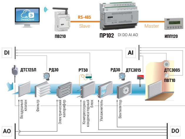
Управление вентиляцией
