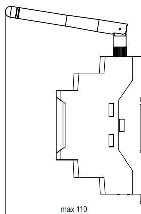
Габаритные размеры Pх210 с антенной
