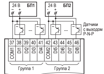
Подключение трехпроводных дискретных датчиков, имеющих выходной транзистор р-п-р-типа с открытым коллектором (для модификаций ПР100-24)
