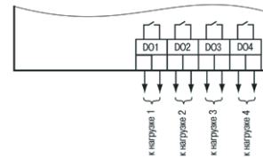
Схема подключения нагрузки к ВЭ типа «Р»
