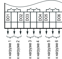
Схема подключения В3 типа «Р»
