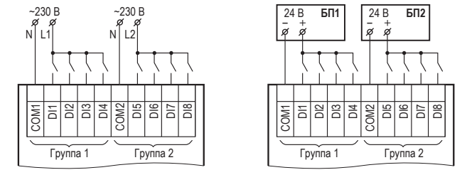
Подключение датчиков типа «сухой контакт» для сигналов =24 В / Подключение датчиков типа «сухой контакт» для сигналов ~230 В
