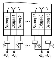
Подключение нагрузки к выходу типа КТ
