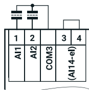
Подключение кондуктометрических датчиков: двухпроводная схема
