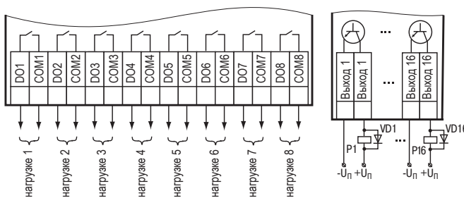
Подключение нагрузки к выходам типа Р / Подключение нагрузки к выходам типа К
