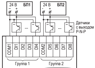
Подключение трехпроводных дискретных датчиков, имеющих выходной транзистор р-п-р-типа с открытым коллектором
