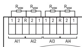
Подключение термометров сопротивления
