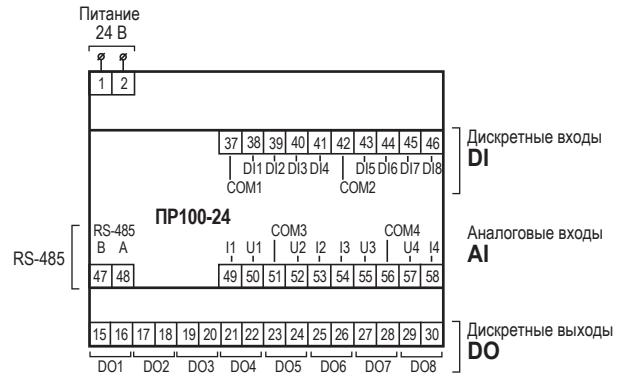
Схема расположения и назначение клемм ПР100-24
