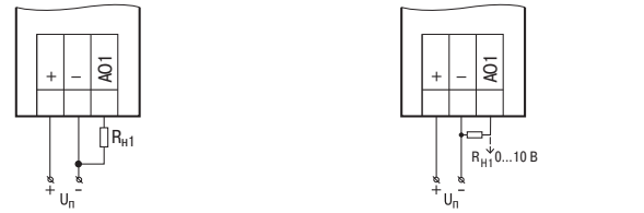
Подключение к аналоговому выходу токовой нагрузки / Подключение к аналоговому выходу нагрузки нагрузки в виде напряжения
