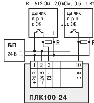
ПЛК100-24, датчик р-р-п-типа
