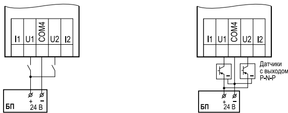
Схема подключения к универсальным входам, работающим в дискретном режиме датчиков типа «сухой» контакт
