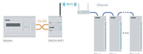
Master в сети Wi-Fi – Slave в сети RS-485
