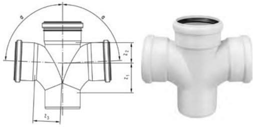
SKDA – крестовина 87°
