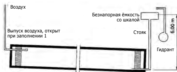
Рис. 10 Проверка герметичности
