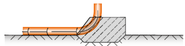
Рис. 9 Фиксация трубопроводов
