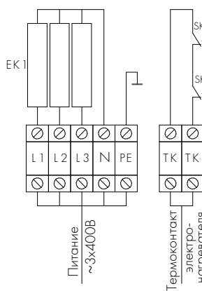
Схема 2. Трехфазное подключение, 1 степень нагрева
