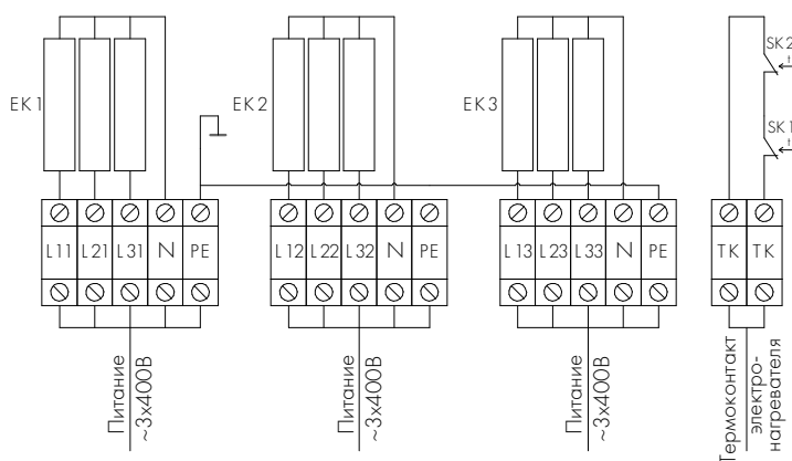
Схема 3. Трехфазное подключение, 2 степени нагрева
