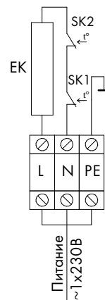
Схема 1. Однофазное подключение, 1 степень нагрева
