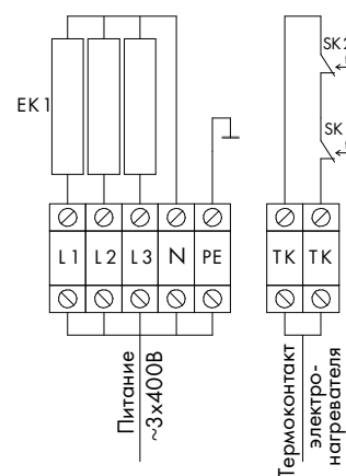
Схема 2. Трехфазное подключение, 1 степень нагрева
