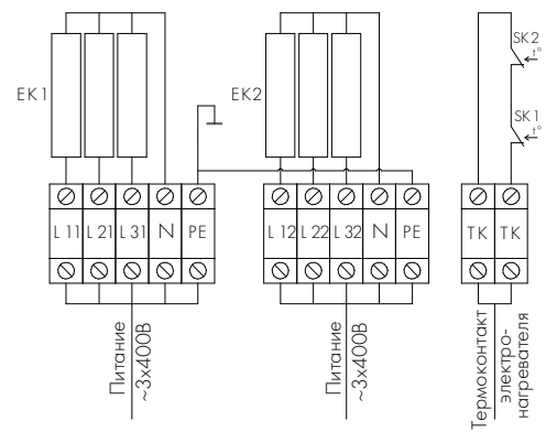
Схема 3. Трехфазное подключение, 2 степени нагрева
