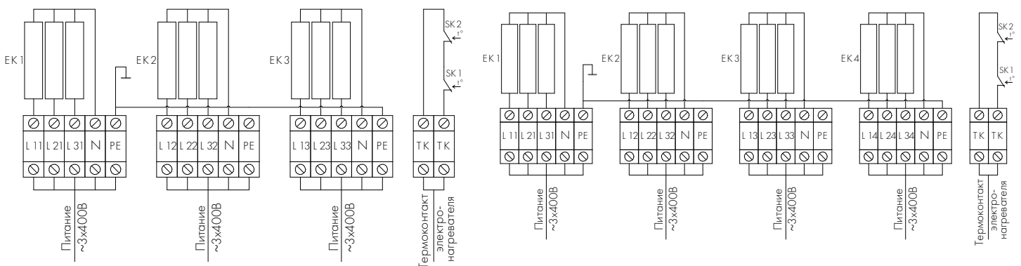
Схема 4. Трехфазное подключение, 3 степени нагрева
