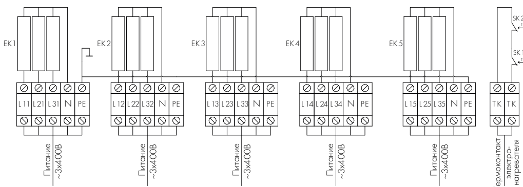
Схема 6. Трехфазное подключение, 5 ступеней нагрева
