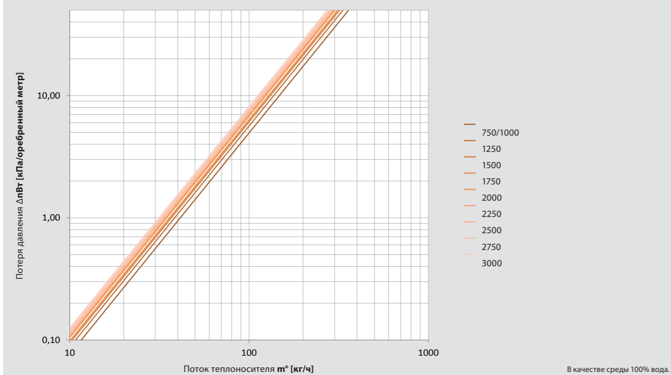
QSKM 195 – без прямого и обратного вентиля
