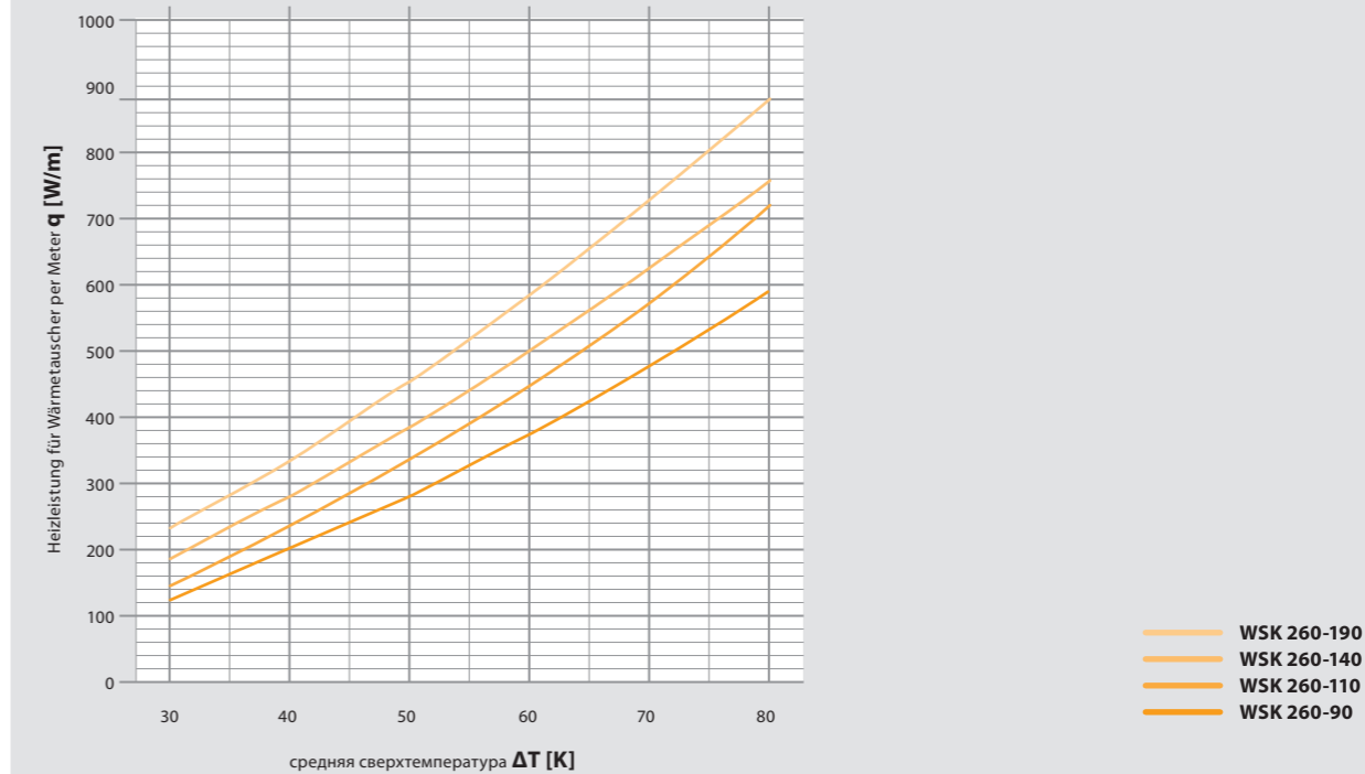
WSK 260 – Ном. теплопроизводительность Q [W] на метр теплообменника
