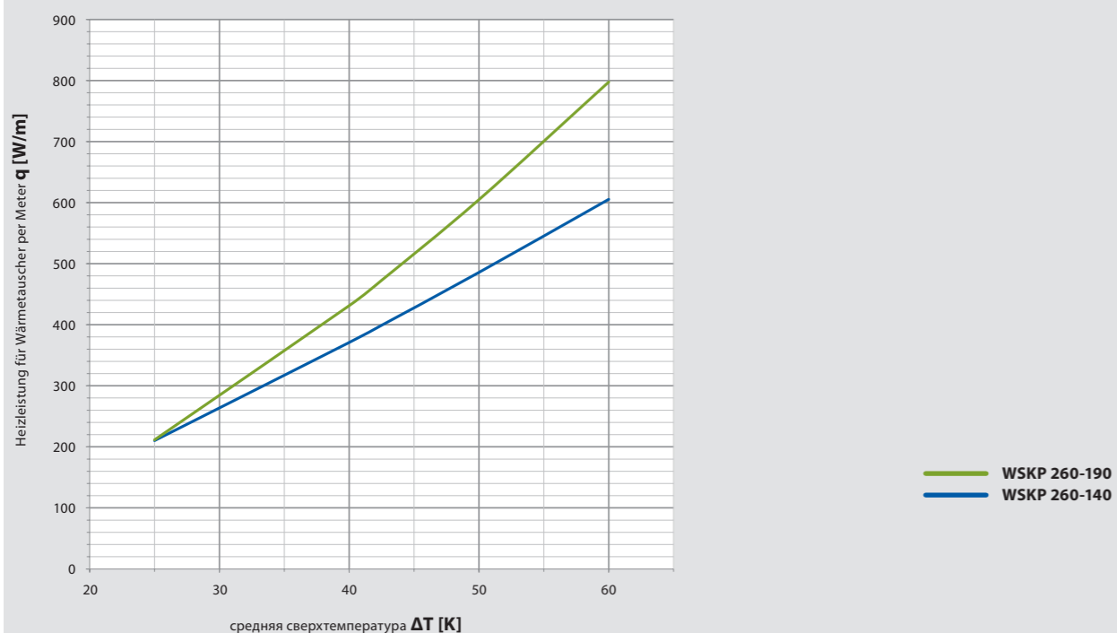
WSKP 260 – Ном. теплопроизводительность Q [W] на метр теплообменника
