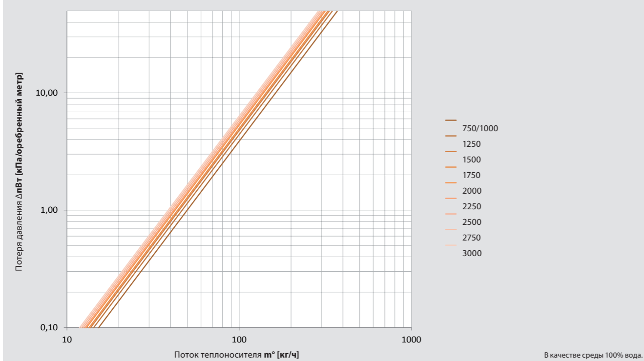
QSKM 195 – без прямого и обратного вентиля
