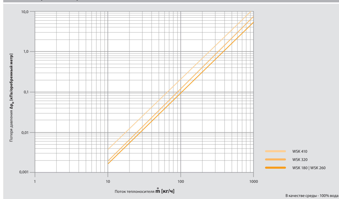
WSK – без прямого и обратного вентиля
