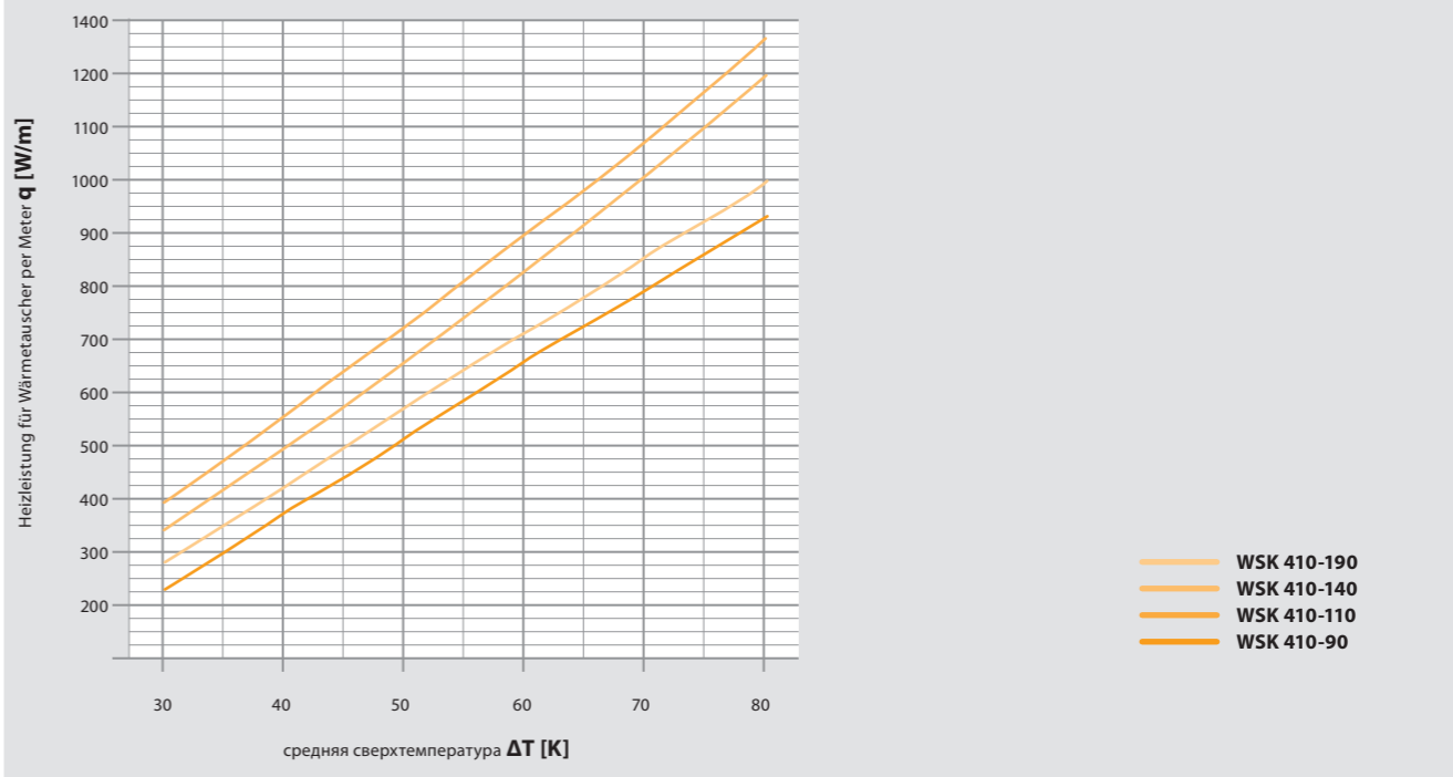
WSK 410 – Ном. теплопроизводительность Q [W] на метр теплообменника
