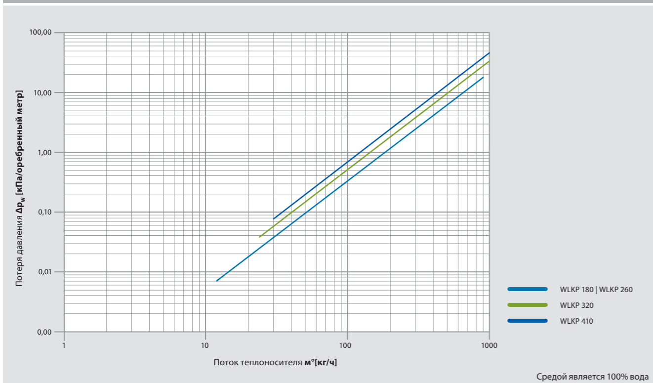
WLKP без подающего и обратного клапана
