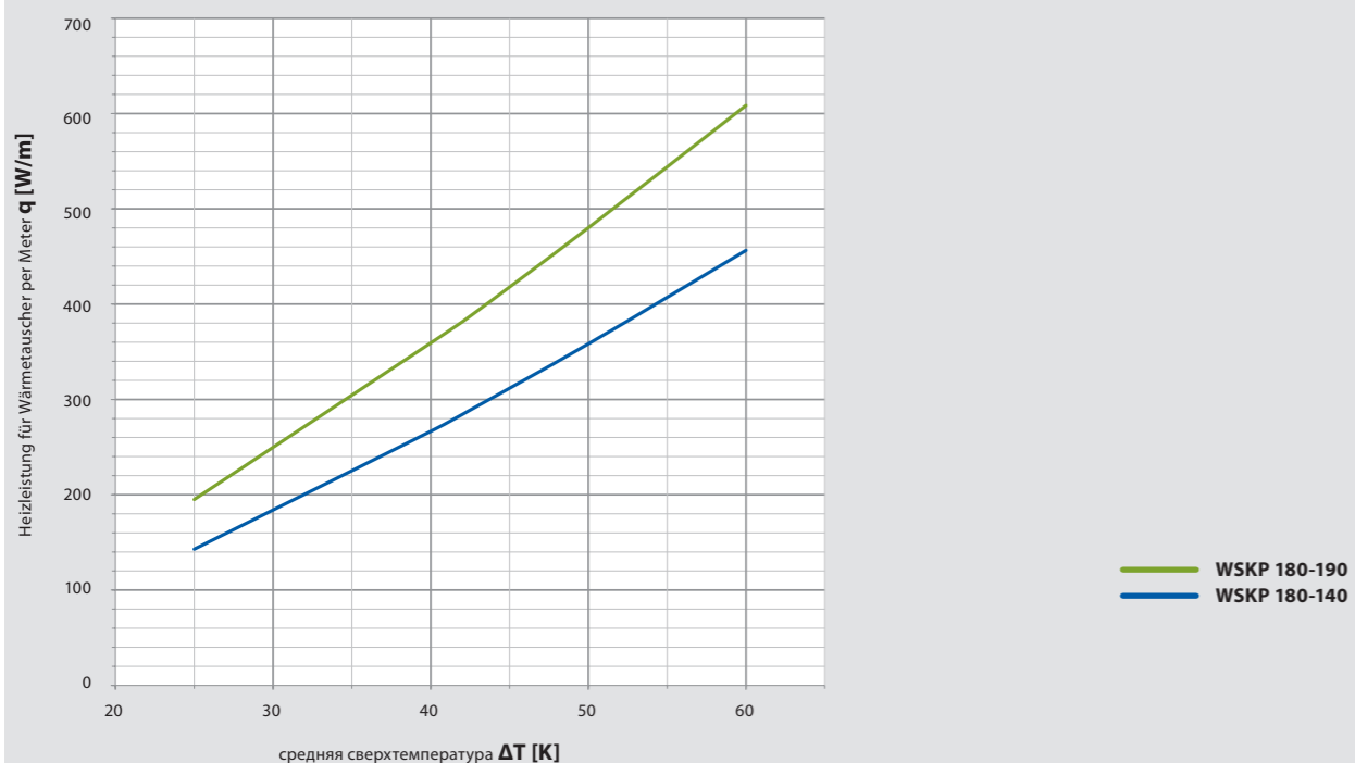
WSKP 180 – Ном. теплопроизводительность Q [W] на метр теплообменника
