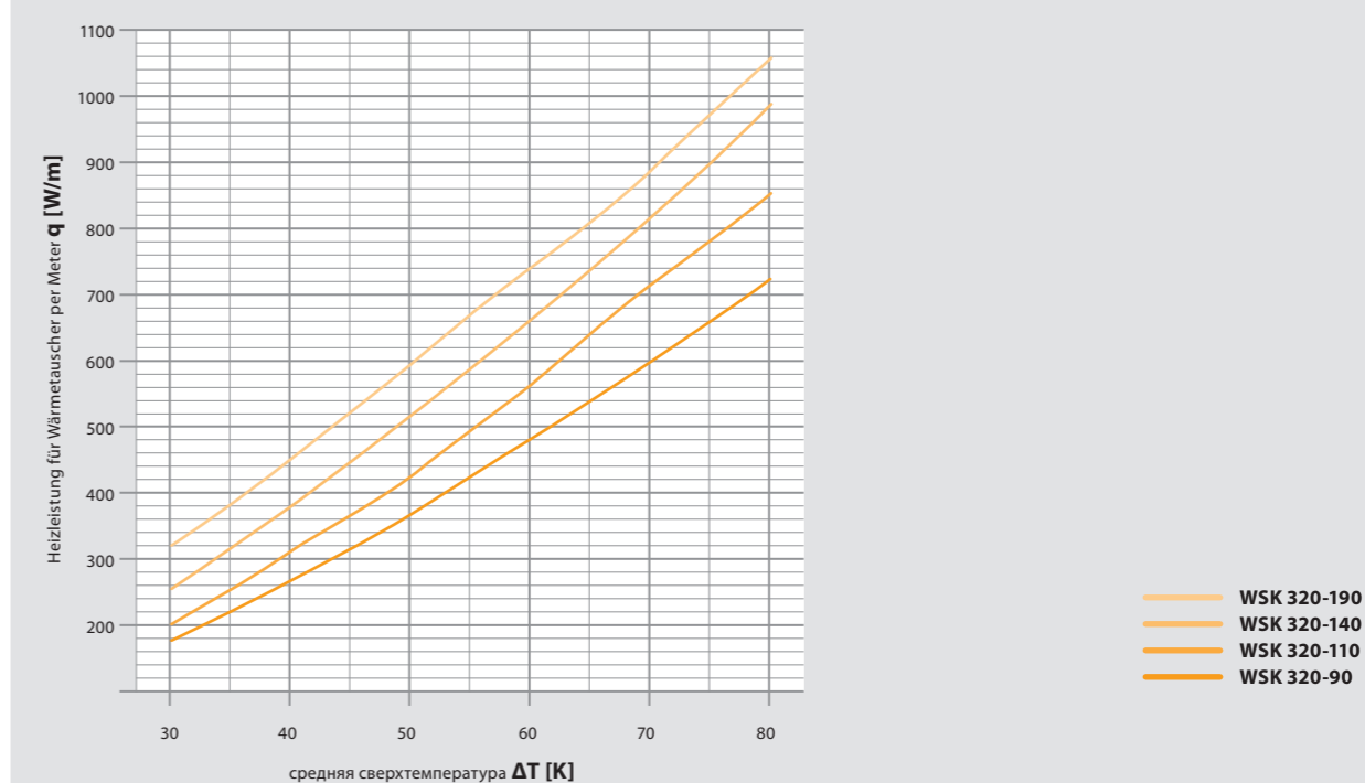
WSK 320 – Ном. теплопроизводительность Q [W] на метр теплообменника
