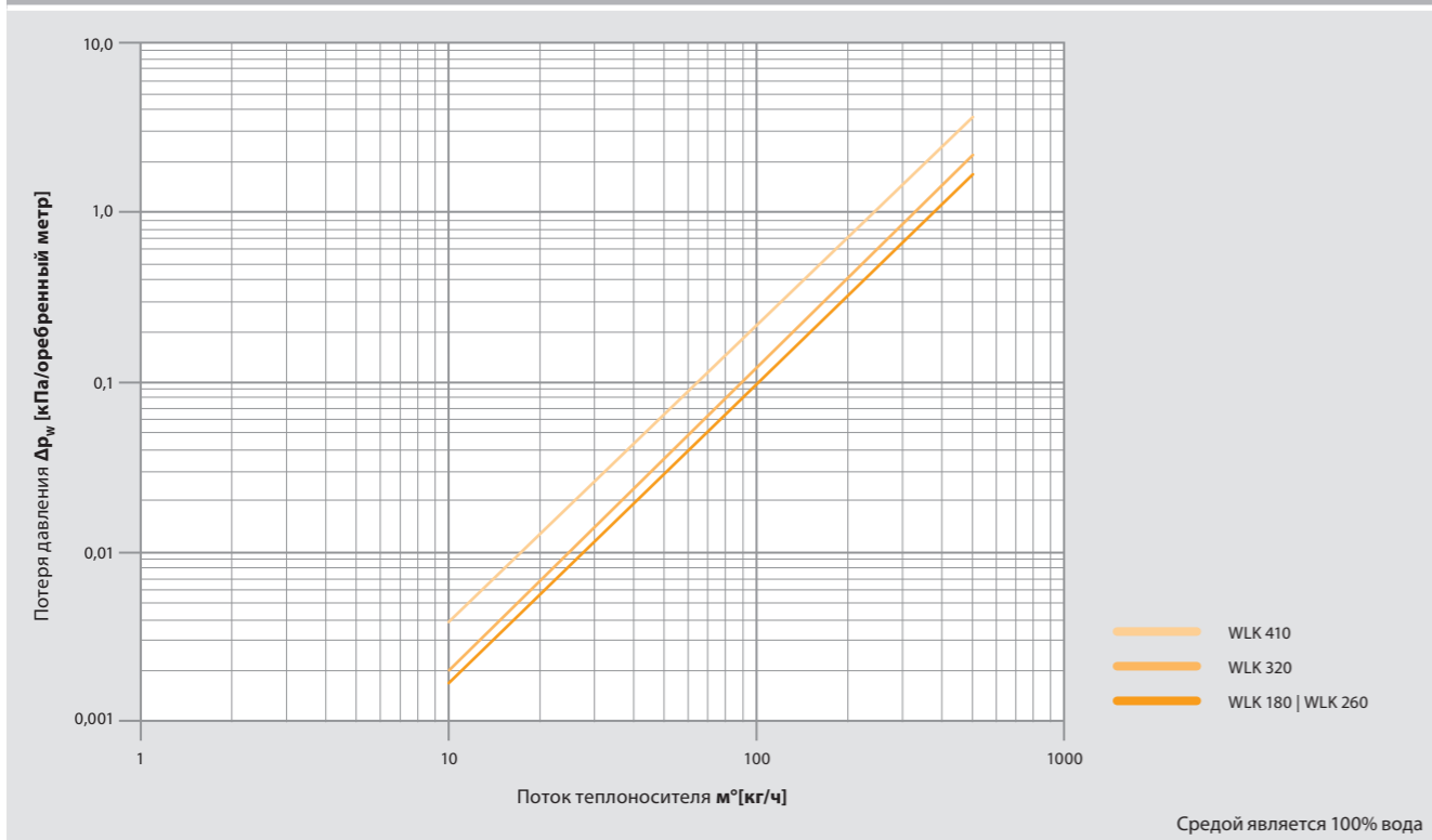
WLK без подающего и обратного клапана
