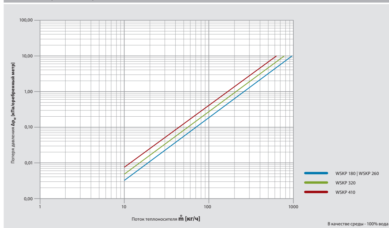
WSKP – без прямого и обратного вентиля
