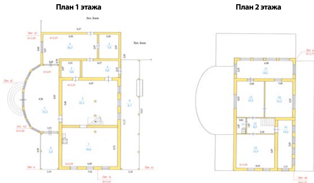
Таб. 2 «РАСЧЕТ ТЕПЛОПТЕРЬ ДОМА»
