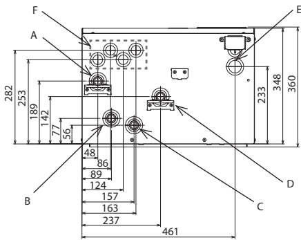
Вид снизу
