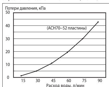
Встроенный теплообменник PUHZ-HW112, 140VNA / YNA2
