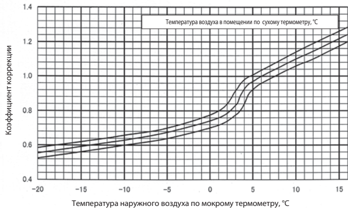
Коррекция теплопроизводительности
