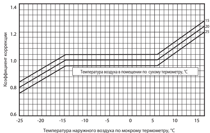
Коррекция теплопроизводительности
