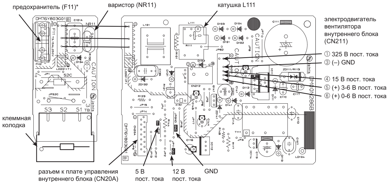
Плата клеммных соединений
