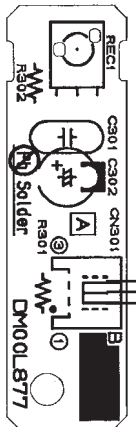
Плата фотоприемника
