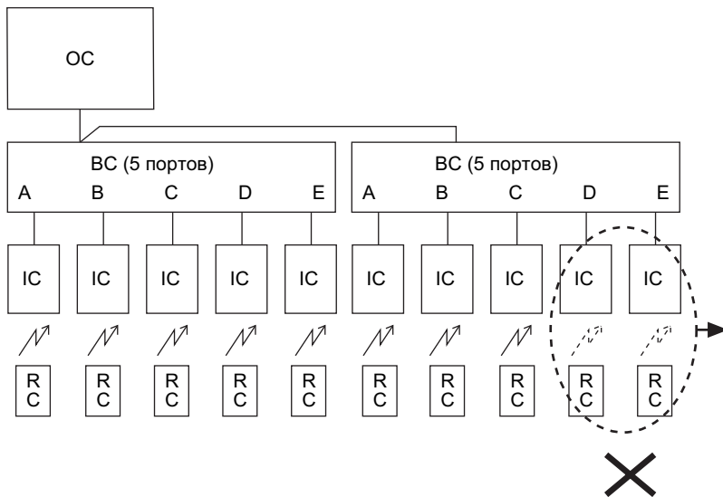
в) два 5-ти портовых ВС (максимум 8 внутренних блоков)
