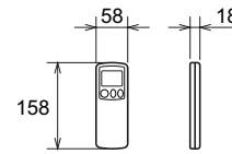
ИК-пульт управления
