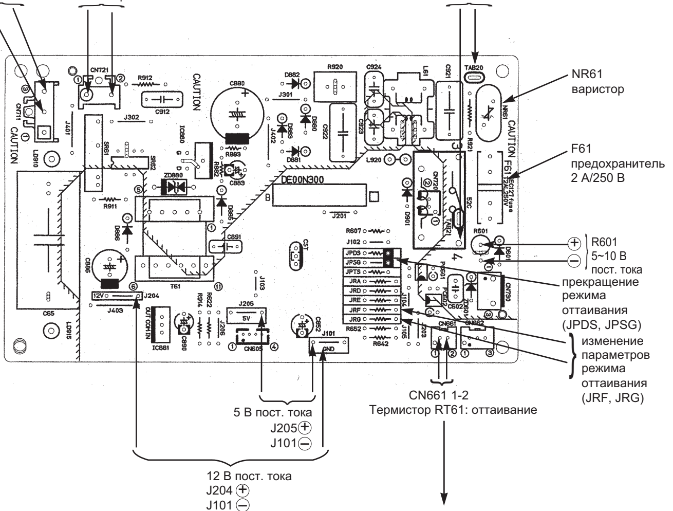
Термистор RT61: оттаивание
