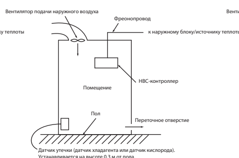
Рис.1-3. Поддача наружного воздуха включается по сигналу датчика утечки.
