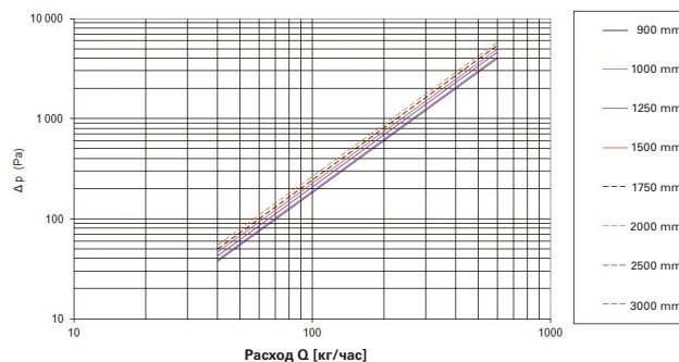
Потери давления теплообменника с 2-мя трубками MINIB SP0 трубка Cu Ø 15 мм
