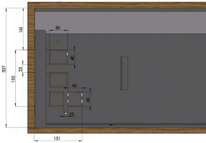
продольное сечение
