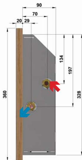
поперечное сечение COIL-KZ 91
