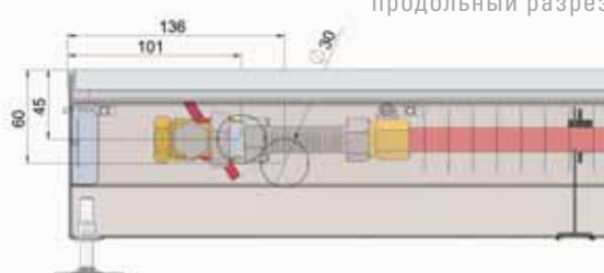
продольный разрез
