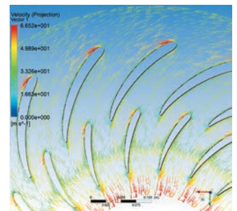
Лопатка, уменьшающая турбулентность
