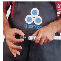
3 Вставка соединителя в трубу
