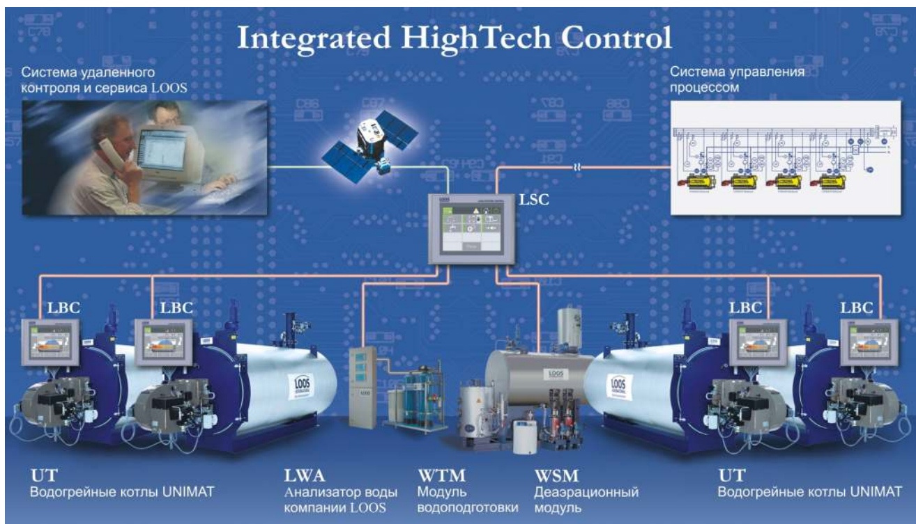
Рис. 8: Система управления котлом и установкой LBC/LSC в составе сложной водогрейной котельной установки
