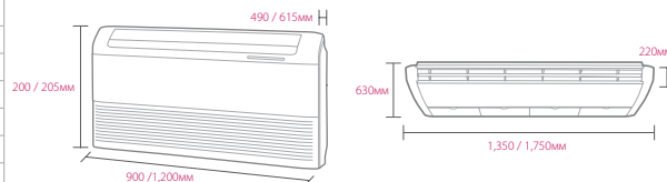
Внутренний блок, габаритные размеры мм
