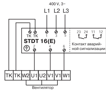
Схема подключения STDT
