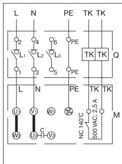
Схема подключения № 2
