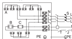
Схема подключения № 3
