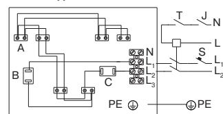
Схема подключения № 2
