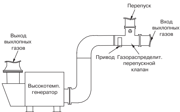
Пример установки газораспределительного перепускного клапана
