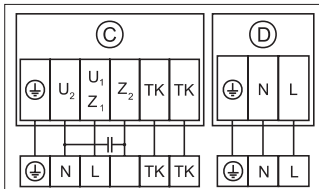
Схема подключения № 4
