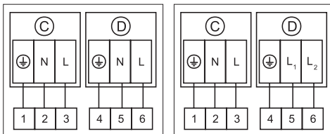
Схема подключения № 1
