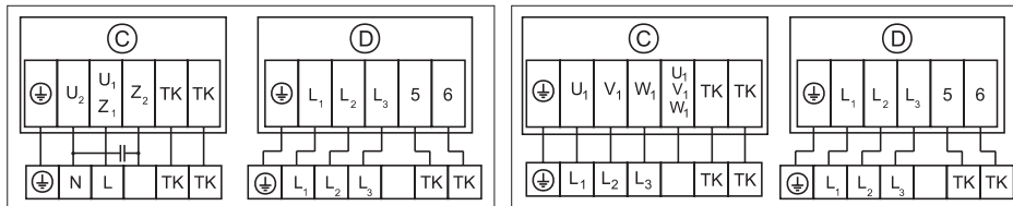
Схема подключения № 12
