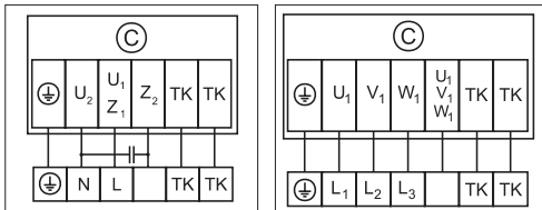
Схема подключения № 14
