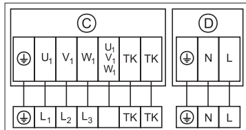
Схема подключения № 5
