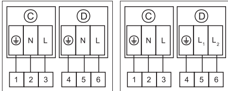
Схема подключения № 1
