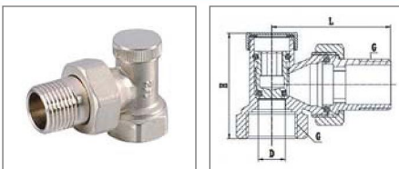
КЛАПАН НАСТРОЕЧНЫЙ УГЛОВОЙ ACS
