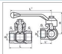
КРАН ШАРОВОЙ, ТРЕХХОДОВОЙ
