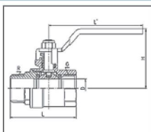
КРАН ШАРОВОЙ MxFL
