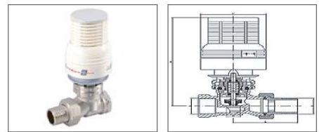
КЛАПАН ПРЯМОЙ С ТЕРМОГОЛОВКОЙ MxTCP
