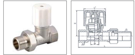
КЛАПАН ПРЯМОЙ FxMCP
