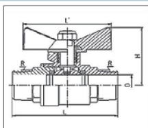
КРАН ШАРОВОЙ MxMB
