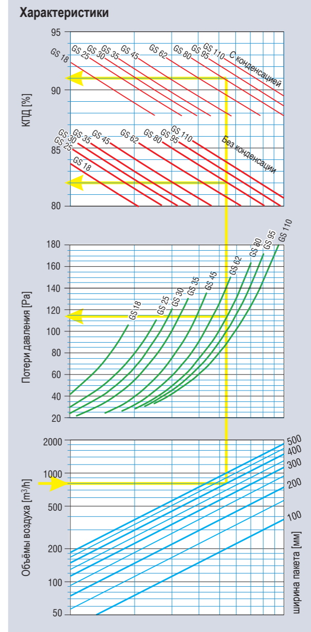
■ Диаграмма рассчитана при одинаковых объёмах наружного и выбрасываемого воздуха
