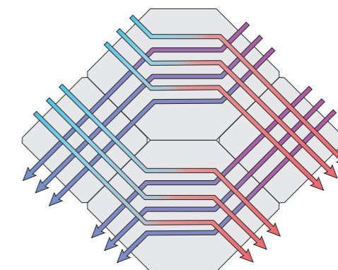
■ Принцип действия комби-теплообменника
